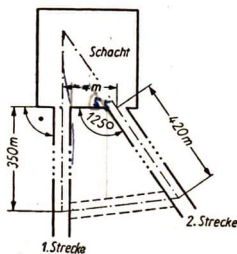
Abb. 55 Grundriß einer Schachanlage
