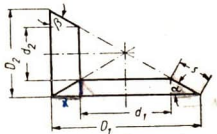
Abb. 27. Kegelräder (schematisch)
