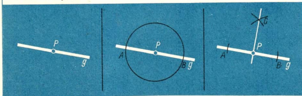
Senkrechte zu g in P
