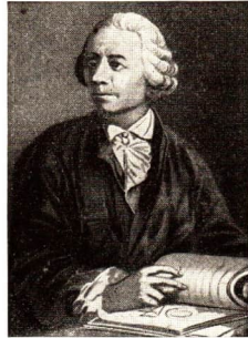
Abb. 3.156. LEONHARD EULER (1707–1783)
