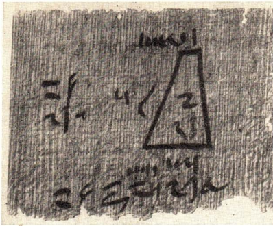
Abb. 3.145. Originaltext der Pyramidenstumpaufgabe des Moskauer Papyrus
