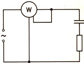
Meßmethode 2
