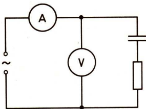
Meßmethode 1
