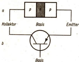
Bild 131/4 a) Aufbau eines Flächentransistors (schematisch), b) Schaltzeichen
