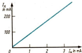
Bild 132/2 Die grafische Darstellung zeigt, daß eine kleine Änderung der Basisstromstärke eine große Änderung der Kollektorstromstärke zur Folge hat.
