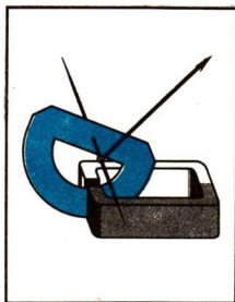
Bild 106/2 Wirbelstromdämpfung bei einem Meßinstrument. Eine Aluminiumscheibe befindet sich zwischen den Polen eines Hufeisenmagneten. Auf diese Weise wird erreicht, daß bei der Messung nicht eine länger dauernde Schwingung stattfindet.
