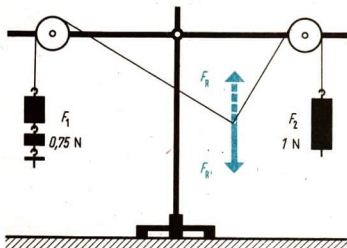
Versuchsaufbau 1 Bild 157/1
