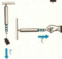
Bild 26/3 Die Längenänderungen der Federn stimmen überein: Gleiche Wirkung, gleiche Kräfte ( F_1 = F_2 ) Bei einem Körper mit der Masse 100 g wird vom Federkraftmesser eine Kraft von etwa 1 N angezeigt.
