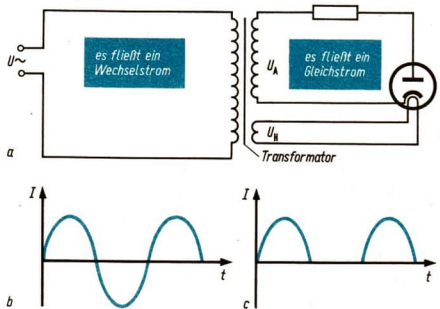
Bild 123/1 Gleichrichterwirkung einer Röhrendiode a) Schaltplan, b) vor dem Gleichrichten, c) nach dem Gleichrichten.
