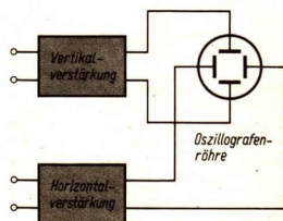
Bild 128/1 Blockschaltbild eines Elektronenstrahloszillografen
