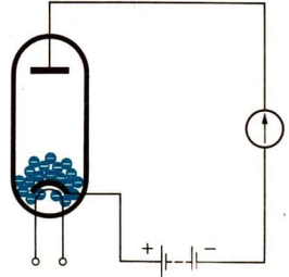
Bild 122/1 Diode in Sperrichtung gepolt.
