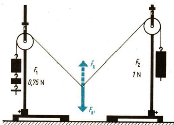
Versuchsaufbau 2 Bild 157/2
