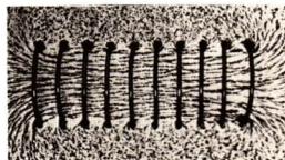
Bild 88/1 Magnetische Feldlinien im Innenraum einer Spule
