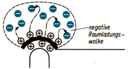
Bild 122/2 Negative Raumladungswolke.
