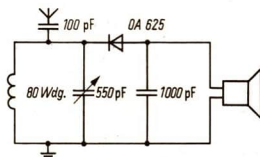
Bild 132/3 Schaltung eines einfachen Rundfunkempfängers mit Diodengleichrichter
