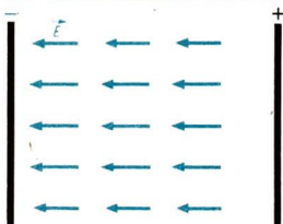
Bild 72/1 Feldstärke im Feld eines Plattenkondensators
