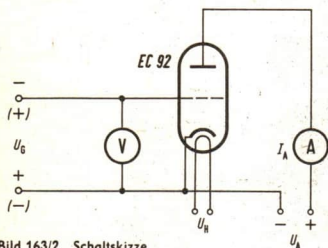
Bild 163/2 Schaltskizze
