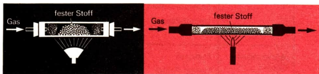
(Rechtes Bild: Apparat für Schülerexperimente)
