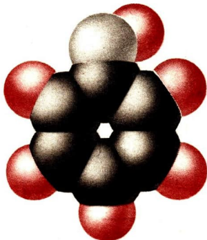
Modell des Phenolmoleküls
