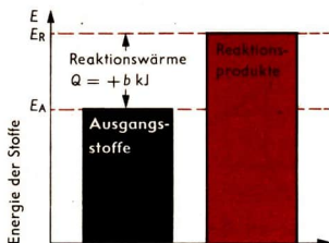
endotherme Reaktion
