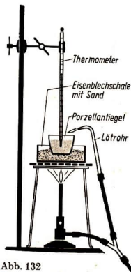
Abb. 132 Flammpunktbestimmung
