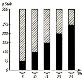
Abb. 71 Seifenverluste von 500 g Seife in 100 l Wasser bei verschiedener Härte
