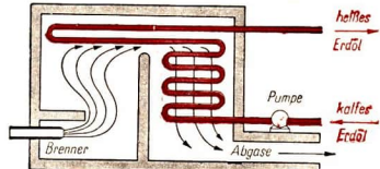
Abb. 16 Schematische Darstellung eines Röhrenofens
