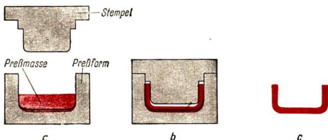
Abb. 100 Schematische Darstellung der Verarbeitung von Preßmassen
