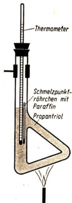
Abb. 130 Schmelzpunktbestimmung von Kerzenparaffin
