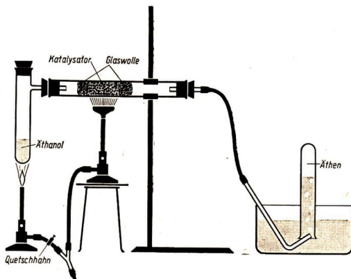
Abb. 129 Darstellung von Äthen aus Äthanol
