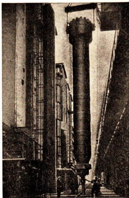
Abb. 30 Sumpffphasekontaktofen der Hydrieranlage im VEB Leuna-Werke „Walter Ulbricht“
