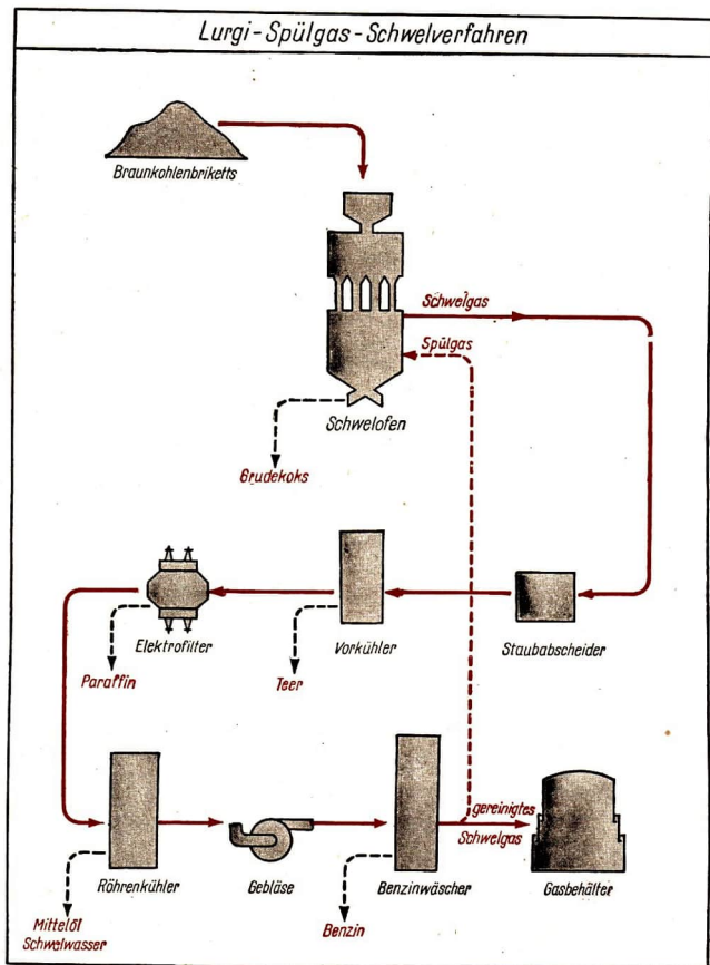
Abb. 29 Schematische Darstellung der Spülgasschwelung nach Lurgi
