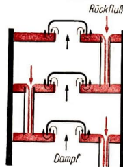
Abb. 17 Fraktioniertürme im VEB Mineralölwerk Lützkendorf
