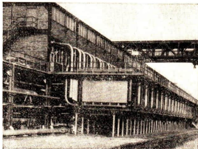
Abb. 33 FISCHER-TROPSCH-Ofenbatterie im VEB Synthesewerk Schwarzheide
