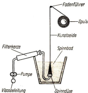
Abb. 112 Spinnen von Viscosefäden (schematische Darstellung)
