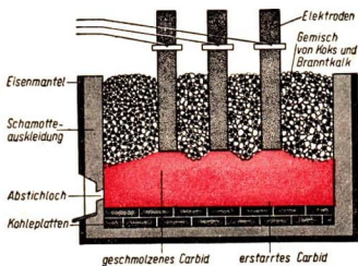
Abb. 11 Schematische Darstellung eines Carbidofens
