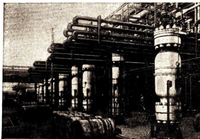
Abb. 42 Teilansicht der Methanolsyntheseanlage im VEB Leuna-Werke „Walter Ulbricht“
