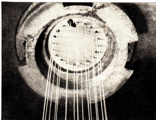
Aus einer Spinnndüse austretende Dederonfäden
