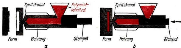
Abb. 95 Schematische Darstellung des Spritzgußverfahrens
