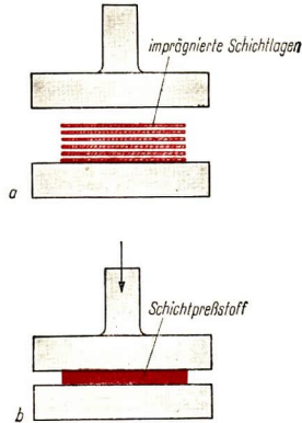
Abb. 106 Schematische Darstellung der Schichtpreßstoffherstellung
