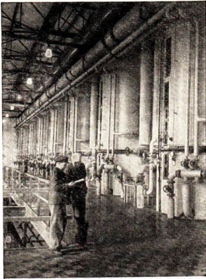
Abb. 81 Verkocherstation im VEB Zuckerfabrik Delitzsch
