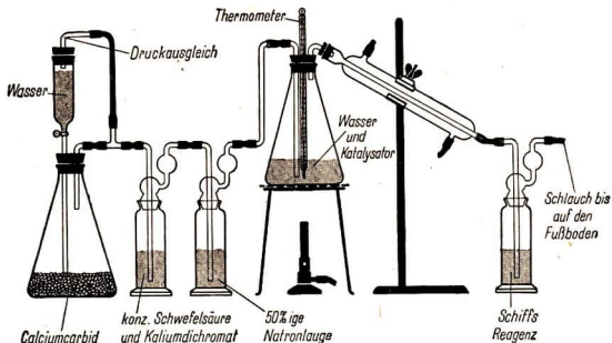
Abb. 47 Darstellung von Äthanal aus Äthin
