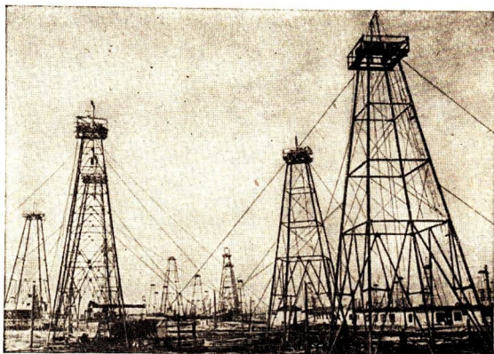
Erdölfeld in der Aserbaidshanischen SSR
