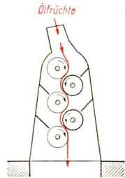
Abb. 55 Schematische Darstellung eines Walzenstuhles
