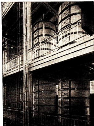
Abb. 45 Destillierkolonnen im VEB Gärungschemie Dessau
