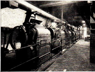
Abb. 54 Walzenstühle für Ölsaaten im VEB Öl- und Fettwerke „Hans Schellheimer“ Magdeburg
