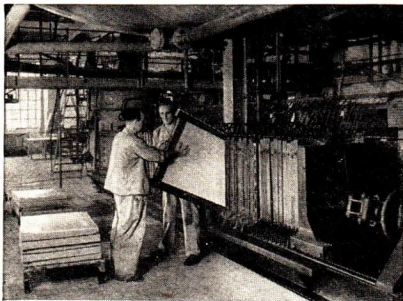
Abb. 66 Kühlpresse in der Konsum-Seifenfabrik Riesa
