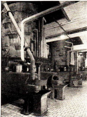
Abb. 56 Preßstation für Ölsaaten im VEB Öl- und Fettwerke „Hans Schellheimer“ Magdeburg
