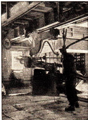
Abb. 10 Abstichöffnung eines Carbidofens im VEB Chemische Werke Buna Schkopau
