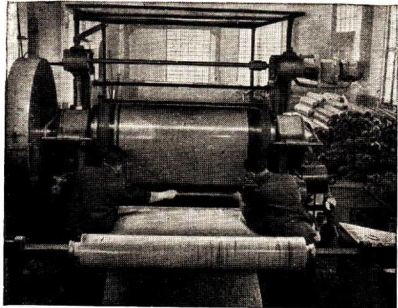
Abb. 92 Kalandern zur Herstellung von PVC-Fußbodenbelag im VEB Elektrochemisches Kombinat Bitterfeld
