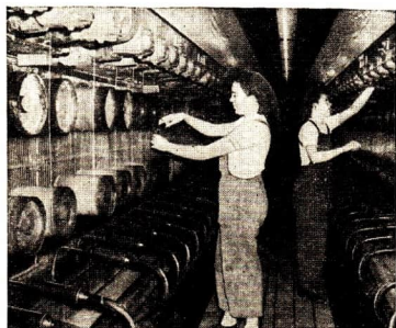
Abb. 111 Zentrifugenspinnmaschine im VEB Chemiefaserwerk „Friedrich Engels“ Premnitz
