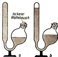
Abb. 134 Äthanolgärung
