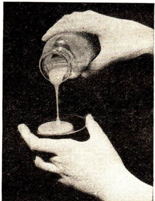
Abb. 110 Viscose
