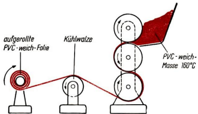
Abb. 93 Schematische Darstellung eines Kalanders
