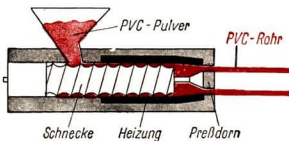
Abb. 90 Schematische Darstellung des Strangpressens von PVC-hart
