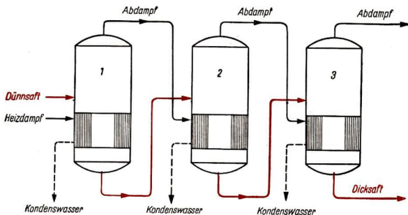
Abb. 80 Schematische Darstellung einer Verdampferstation
