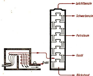
Abb. 19 Destillation des Erdöls (schematische Darstellung)
