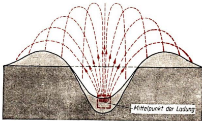
Abb. 126 Trichtersprengung
