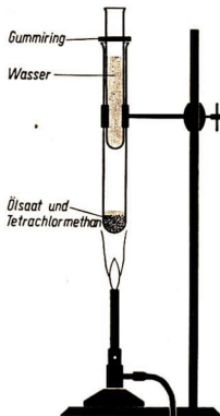
Abb. 136 Extraktion von Ölsaat
