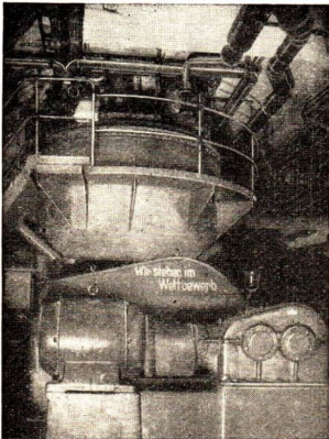
Abb.109 Xanthogenatkneter im VEB Thüringisches Kunstfaserwerk „Wilhelm Pieck“ Schwarzra
