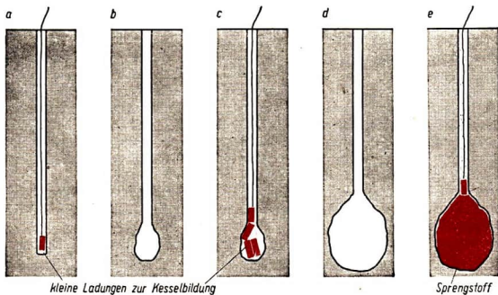
Abb. 124 Kesselladung
