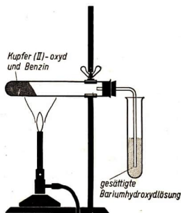
Abb. 128 Nachweis von Kohlenstoff in Benzin
