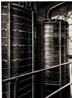
Abb. 91 Waschtürme aus PVC-hart-Platten in der Schwefelsäurefabrik des VEB Chemiefaserwerk „Friedrich Engels“ Premnitz
