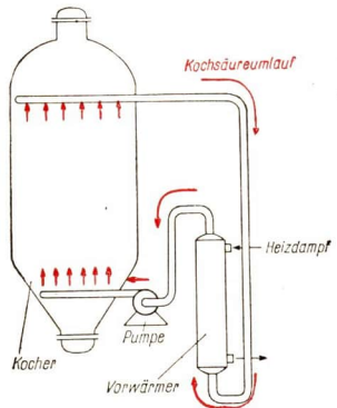
Abb. 86 Schematische Darstellung eines Zellstoffkochers
