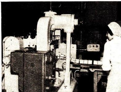
Abb. 60 Verpackungsmaschine für Margarine im VEB Berolina Margarinefabrik Berlin
