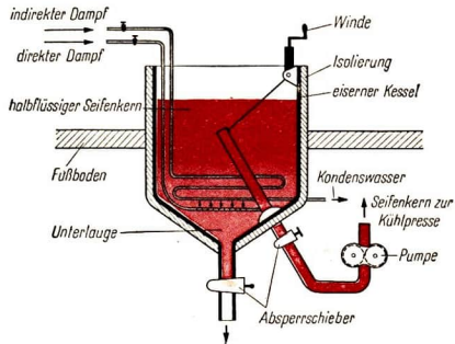
Abb. 65 Schematische Darstellung eines Siedekessels
