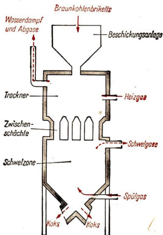
Abb. 28 Schematische Darstellung eines Schwelofens
