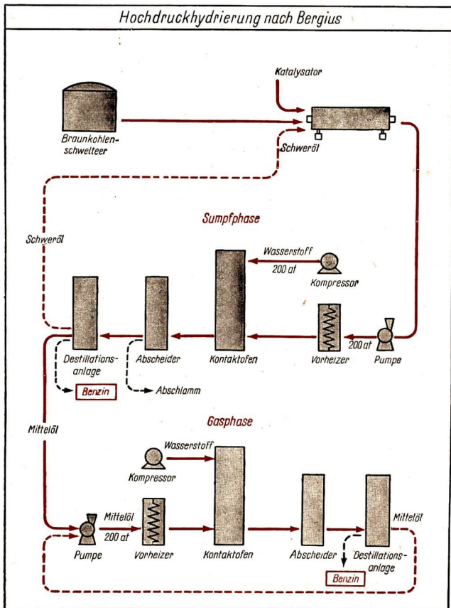
Abb. 32 Schematische Darstellung der Hochdruckhydrierung nach Bergius
