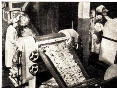
Abb. 68 Piliermaschine im VEB Patina Seifen- und Parfümeriefabrik Halle
