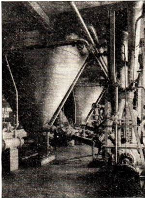
Abb. 85 Unterteil eines Zellstoffkochers im VEB Filmfabrik Agfa Wolfen
