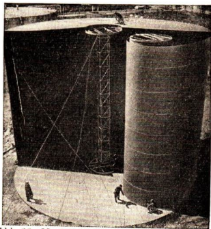
Abb. 26 Montage von Erdöltanks aus vorgefertigten Großteilen in der Sowjetunion
