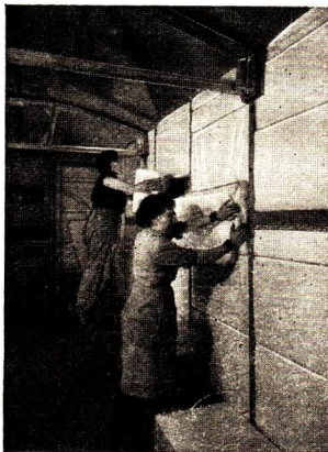
Abb. 104 Auskleiden eines Kühlwagens mit Piatherm im VEB Waggonbau Dessau Zum Schutz gegen Feuchtigkeit sind die Piathermplatten mit Perfol eingeschlagen.
