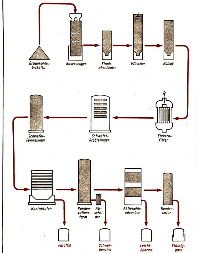
Abb. 35 Schematische Darstellung des FISCHER-TROPSCH-Verfahrens
