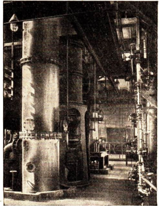
Abb. 48 Äthansäure-Kontakanlage im VEB Chemische Werke Buna, Schkopau
