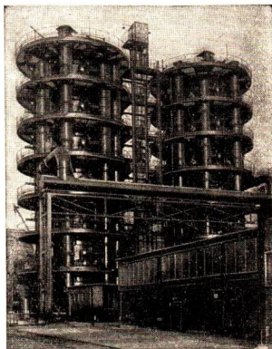
Abb. 34 Aktivkohleadsorber zur Benzingewinnung im VEB Synthesewerk Schwarzheide
