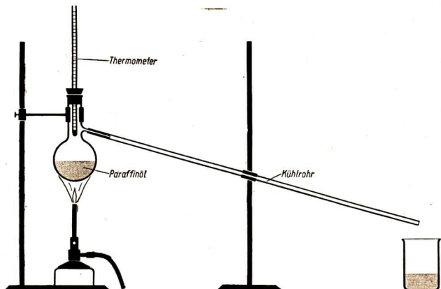
Abb. 131 Destillation von Paraffinöl
