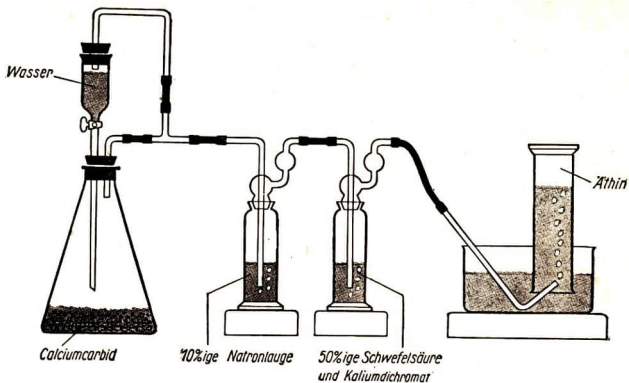
Abb. 13 Herstellung von Äthin aus Calciumcarbid
