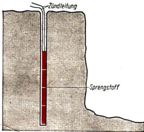
Abb. 125 Säulenladung
