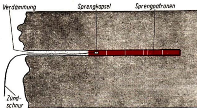
Abb. 123 Sprengladung in einem Bohrloch
