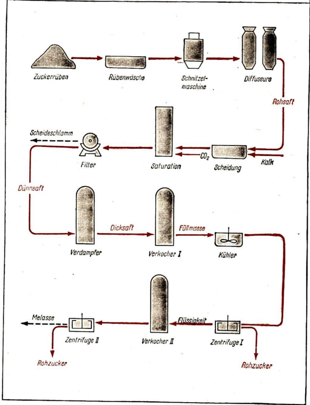
Abb. 83 Schematische Darstellung der Rohzuckergewinnung
