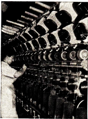
Abb. 116 Maschine zum Verstrecken und Zwirnen von Dederonseide
