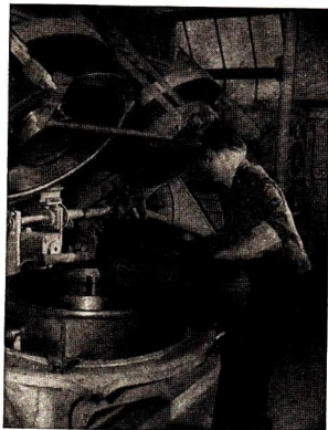
Abb. 99 Vulkanisierkessel für Flugzeugreifen im VEB Reifenwerk Fürstenwalde
