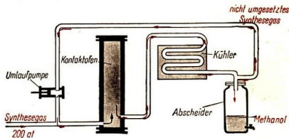
Abb. 43 Schematische Darstellung einer Methanolsyntheseanlage
