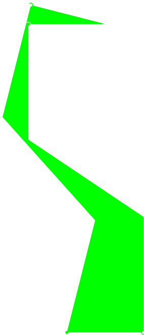
Abb. 4: zweite Modifikation des Vorderbergschen Neunecks
