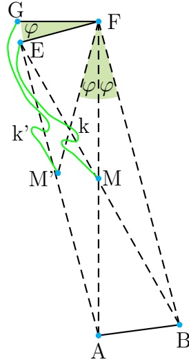
Abb. 20: Grundgerüst des Vorderbergteils mit beliebiger Randkurve
