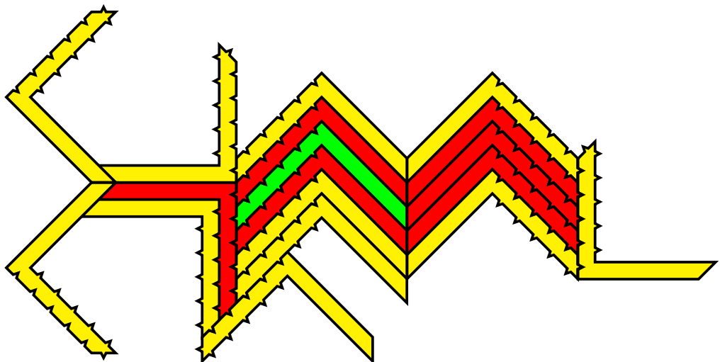
Abb. 13: Teil mit Heesch-Zahl 2
