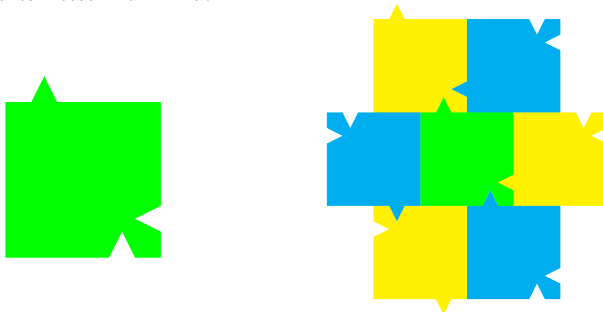
Abb. 11: einfaches Teil mit Heesch-Zahl 1 und dessen Umschließung
