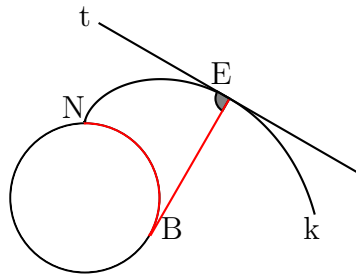
Abb. 23: Konstruktion einer Kreisevolvente
