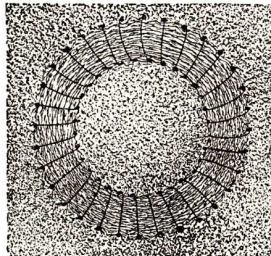
Abb. 47. Feld einer Ringspule
