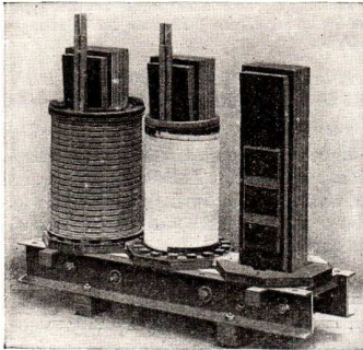
Abb. 138. Dreiphasenstromtransformator
