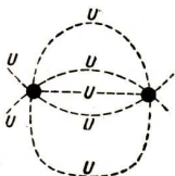
Abb. 56. Gleiche Spannung längs verschiedener elektrischer Feldlinien
