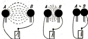
Abb. 15. Spannung und Feldlinienlänge
