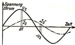
Abb. 132. Zur Berechnung der Arbeitsleistung eines phasenverschobenen Wechselstroms
