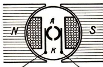
Abb. 108. Schnitt durch die Dynamomaschine von W. von Siemens
