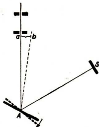
Abb. 249. Bestimmung der Lichtgeschwindigkeit durch Foucault
