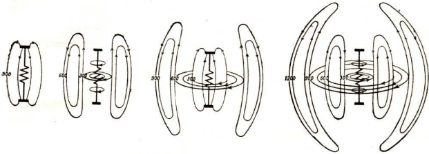
Abb. 307. Ausbreitung des Feldes eines Dipols
