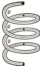
Abb. 88. Die in mehreren Drahtwindungen induzierte Spannung
