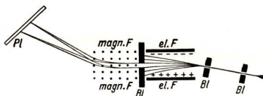
Abb. 152. Kanalstrahlenverlauf im Massenspektograph
