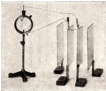
Abb. 31. Versuche zur Influenz
