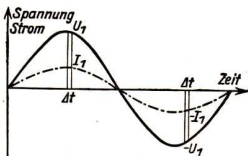
Abb. 131. Zur Berechnung der Arbeit eines phasengleichen Wechselstroms
