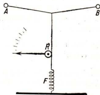
Abb. 3. Hitzdrahtinstrument (schematisch)
