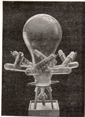
Abb. 179. Quecksilberdampfgleichrichter
