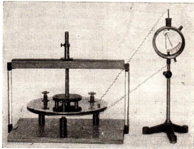
Abb. 18. Spannung und Feldlinienlänge im homogenen Feld
