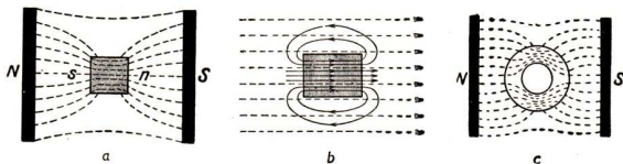
Abb. 65. Eisen im Magnetfeld
