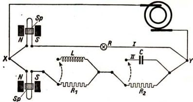
Abb. 126. Nachweis der Phasenverschiebung von Wechselströmen
