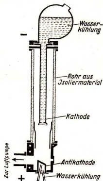
Abb. 349. Moderne Röntgenröhre
