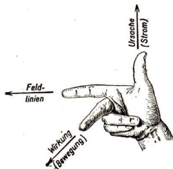
Abb. 73. Dreifingerregel
