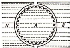
Abb. 100. Feldlinien in einer Dynamomaschine
