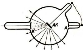
Abb 150. Röntgenröhre alter Bauart
