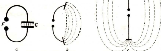
Abb. 305. a geschlossener, b halboffener, c offener Schwingungskreis
