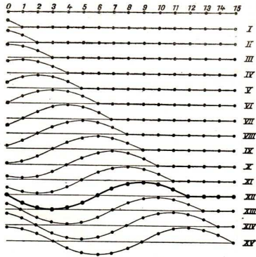
Abb. 201. Bildung einer fortschreitenden Querverwelle
