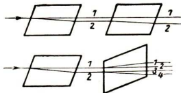
Abb. 277. Wiederholter Durchgang des Lichtes durch Kalkspat
