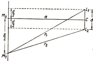
Abb. 255. Bestimmung der Wellenlänge des Lichtes nach Fresnel
