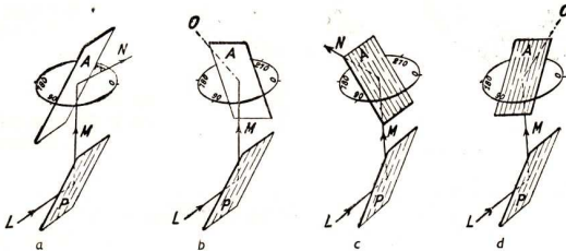
Abb. 278. Polarisation des Lichtes durch Reflexion
