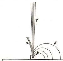
Abb. 182. \alpha -, \beta - und \gamma -Strahlung einer Radiumverbindung ( R )
