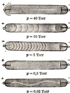
Abb. 165. Leuchten in Röhren bei verschiedenen Gasdrucken
