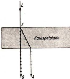
Abb. 285. Ordentlicher und außerordentlicher Strahl bei der Doppelbrechung des Lichtes im Kalkspat
