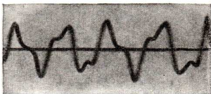
Abb. 212. Überlagerte Schwingungen eines Sandpendels
