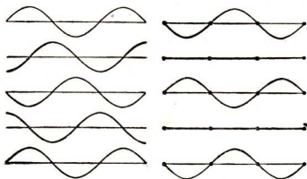
Abb. 224. Schwingungszustände einer fortschreitenden und einer stehenden Welle
