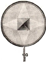
Abb. 279. Nichtpolarisiertes Licht
