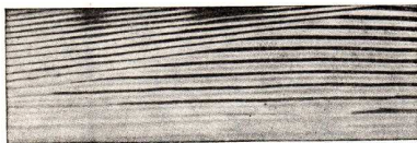
Abb. 246. Brechung von Wasserwellen
