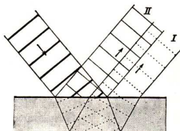
Abb. 259. Reflexion am dünnen Blättchen. Wellenverlauf
