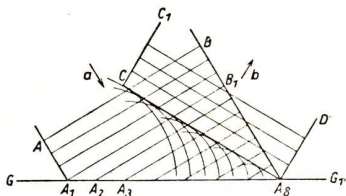
Abb. 240. Reflexion nach dem Huygensschen Prinzip
