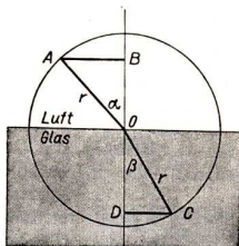
Abb. 250. Brechungsgesetz
