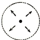
Abb. 195. Ausbreitung eines Impulses im Innern eines elastischen Körpers
