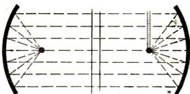
Abb. 345. Ausbreitung der Wärmestrahlen
