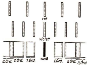
Abb. 274. Beugungsstreifen und Beugungsspektrum
