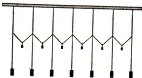
Abb. 196. Entstehung einer Welle aus einer Schwingung
