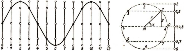
Abb. 204. Wellenlinie bei harmonischer Erregung der Welle
