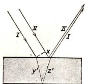
Abb. 258. Reflexion am dünnen Blättchen. Strahlenverlauf
