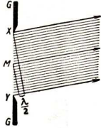
Abb. 269. Erklärung der Entstehung der ersten seitlichen dunklen Streifen
