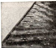
Abb. 236. Reflexion von Wasserwellen
