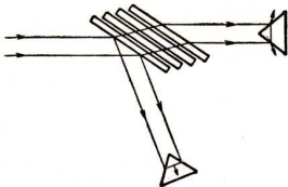
Abb. 281. Polarisation des Lichtes durch Brechung
