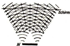
Abb. 266. Entstehung der Beugungsbilder hinter einem Hindernis
