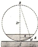
Abb. 263. Erklärung der Newtonschen Ringe
