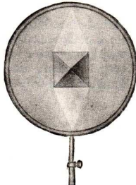
Abb. 280. Polarisiertes Licht
