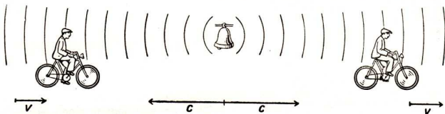
Abb. 207. Dopplersches Prinzip
