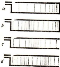
Abb. 229a—d. Stehende Wellen in Pfeifen
