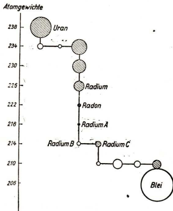
Abb. 353. Der radioaktive Zerfall des Urans
