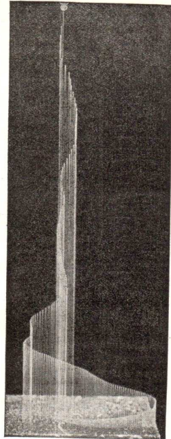
Abb. 191. Wiederholter Fall einer Stahlkugel auf eine Glasplatte
