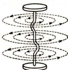
Abb. 321. Magnetische Wellen
