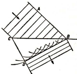
Abb. 247. Brechung nach dem Huygensschen Prinzip
