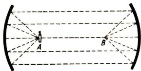
Abb. 239. Reflexion von Schallwellen
