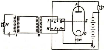
Abb. 177. Versuch zur Lautverstärkung eines Fernsprechstromes
