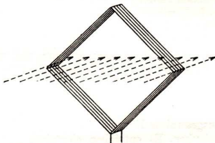
Abb. 323. Rahmenantenne
