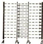
Abb. 37. Das Gegenfeld der influenzierten Ladungen
