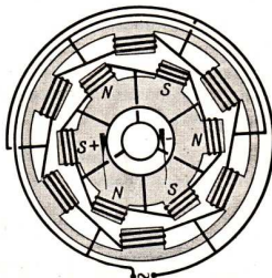
Abb. 117. Schaltung einer sechsspuligen Wechselstromdynamomaschine
