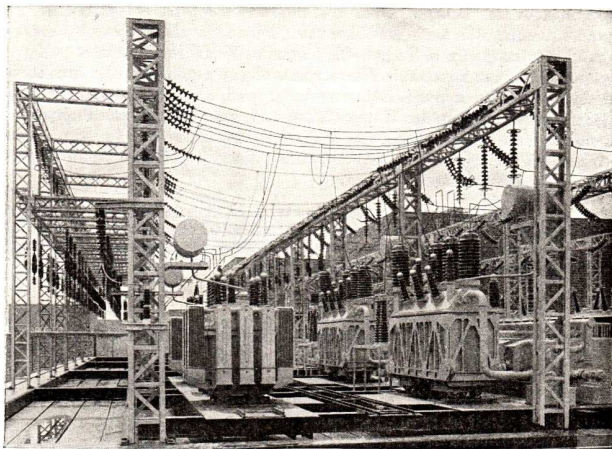
Abb. 139. Umspannwerk
