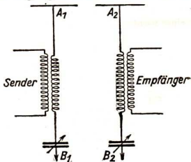
Abb. 315. Antennenkreise von Sender und Empfänger
