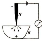
Abb. 172. Kristalldetektor, schematisch
