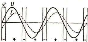
Abb. 134. Positive Leistung eines Wechselstroms geringer Phasenverschiebung
