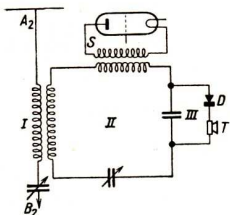
Abb. 324. Überlagerungsempfang bei drahtloser Telegraphie
