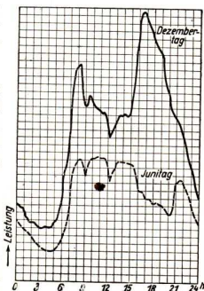
Abb. 140. Belastungskurve eines Elektrizitätswerkes
