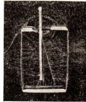
Abb. 17. Feldlinienbild des Elektroskops
