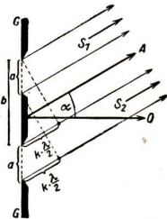
Abb. 273. Beugung am Doppelspalt
