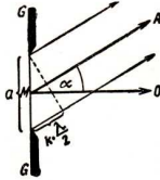
Abb. 271. Zusammenhang zwischen Beugungswinkel, Spaltbreite und Wellenlänge
