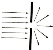
Abb. 243. Beugung nach dem Huygensschen Prinzip
