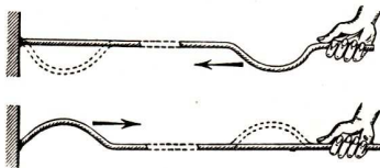
Abb. 221. Reflexion einer Halbwellen an einer festen Wand
