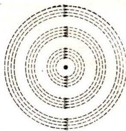
Abb. 322. Magnetischer Wellenzug
