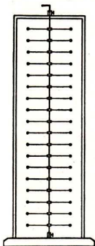
Abb. 194. Reflexion eines Drehimpulses
