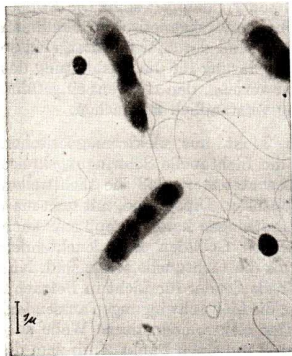
Abb. 348. Paratyphusbakterien Elektronenoptische Vergrößerung 6500 : 1
