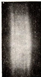
Abb. 252. Fresnelscher Streifen
