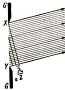
Abb. 270. Erklärung der Entstehung der ersten seitlichen hellen Streifen
