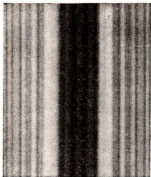
Abb. 265. Beugungstreifen hinter einem dünnen Draht
