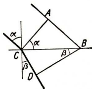
Abb. 248. Brechungsgesetz
