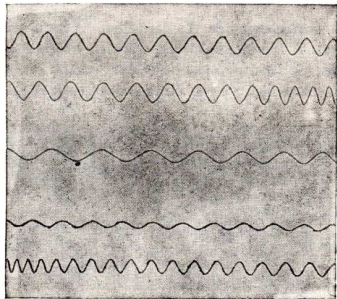
Abb. 205. Stimmgabelschwingungen
