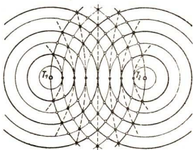
Abb. 217. Interferenz von Schallwellen
