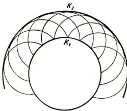
Abb. 233. Elementarwellen und Frontwelle
