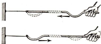
Abb. 220. Reflexion einer Halbwellen an einem freien Ende
