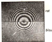
Abb. 261. Newtonsche Ringe im roten und blauen Licht
