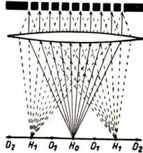
Abb. 272. Beugung am Gitter
