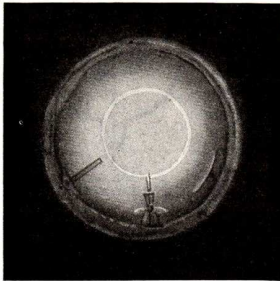
Abb. 149. Elektronenring im Magnetfeld
