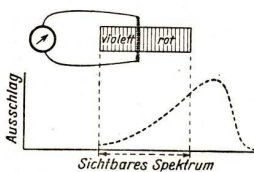
Abb. 344. Energieverteilung im Spektrum
