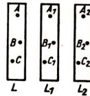
Abb. 257. Kohärentes Licht
