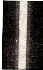
Abb. 268. Beugung am schmalen Spalt
