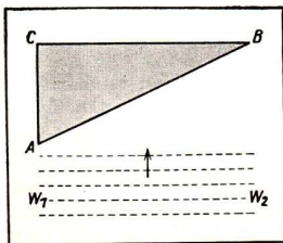
Abb. 245. Schema der Brechung von Wasserwellen
