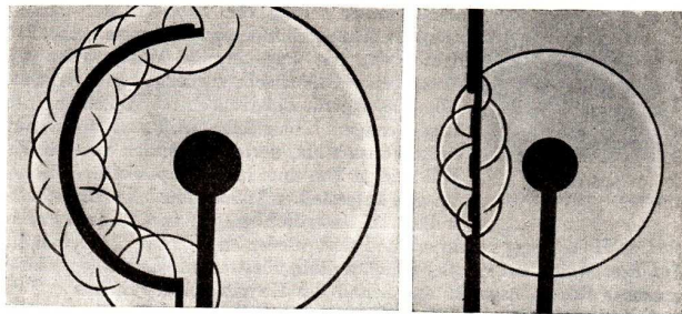
Abb. 234. Elementarwellen und Frontwelle bei Schallwellen nach Foley und Souder
