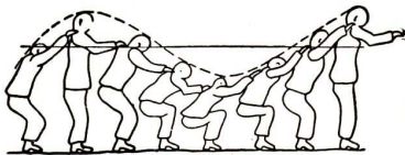
Abb. 200. Veranschaulichung einer Welle
