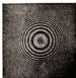
Abb. 260. Newtonsche Ringe im Natriumlicht
