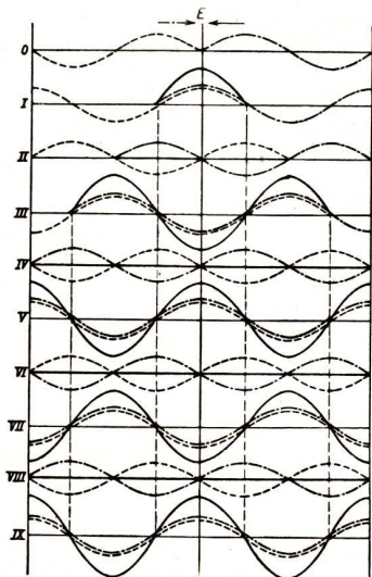
Abb. 223. Bildung einer stehenden Welle
