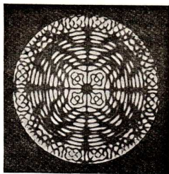
Abb. 227. Stehende Welle im Innern eines vollen Glaszylinders
