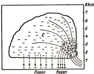
Abb. 186. Elektrisches Feld einer Gewitterwolke
