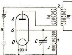
Abb. 298. Schaltung eines Senders
