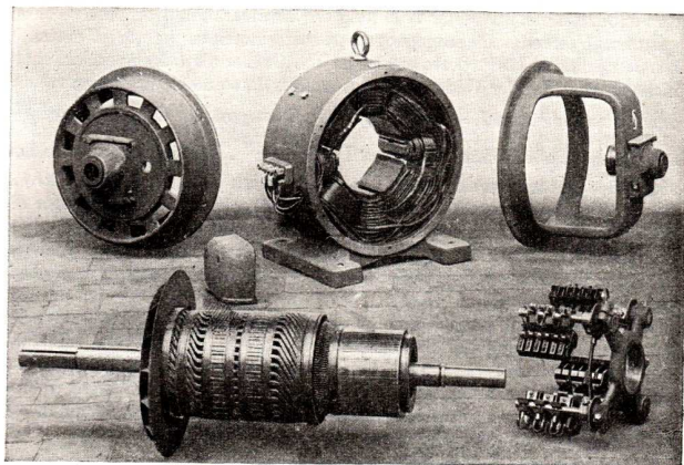
Abb. 115. Teile des Gleichstrommotors
