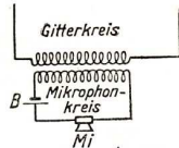
Abb. 325. Übertragung des Mikrophonwechselstroms bei drahtloser Telephonie
