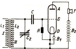
Abb. 300. Verstärkung und Gleichrichtung einer hochfrequenten Schwingung
