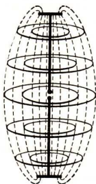
Abb. 306. Das elektromagnetische Feld eines Dipols
