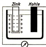
Abb. 144. Galvanisches Element
