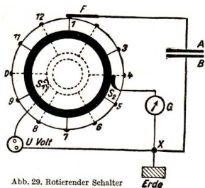
Abb. 29. Rotierender Schalter
