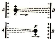
Abb. 133. Geladener Körper im Wechselfeld
