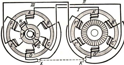
Abb. 118. Drehstromdynamomaschine und -motor
