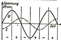
Abb. 135. Strom mit 90^\circ Phasenverschiebung leistet keine Arbeit
