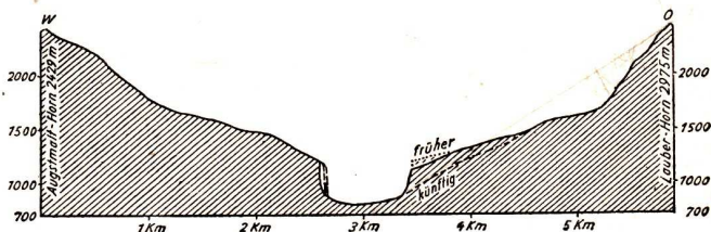
Abb. 1. Überhöhter Querschnitt durch das Tal des Lütschine. Eingesenkter Gletschertrog (nach G. Wagner)
