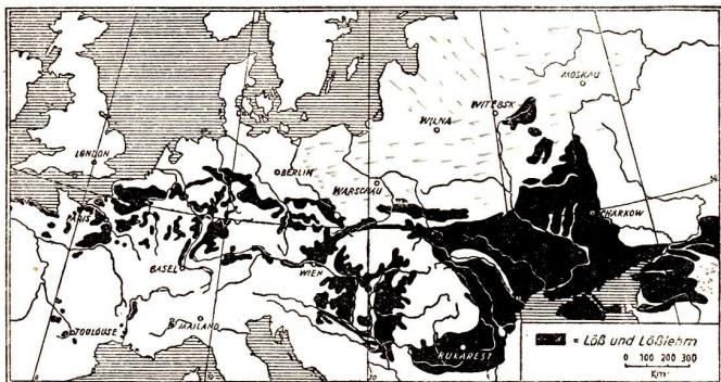
Abb. 4. Verbreitung des Lößes in Europa (nach R. Grahmann)
