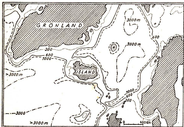
Abb. 5. Tiefenkarte des Nordatlantik mit dem Wyville-Thomson-Rücken (nach W. Wundt)
