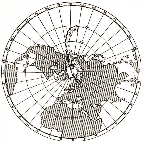
Abb. 6. Die Wanderung des Nordpols von der Vergangenheit vor über 300 Millionen Jahren bis in die Zukunft. Die angeschriebenen Zahlen bedeuten jeweils 10 Millionen Jahre (nach M. Milankovitch)
