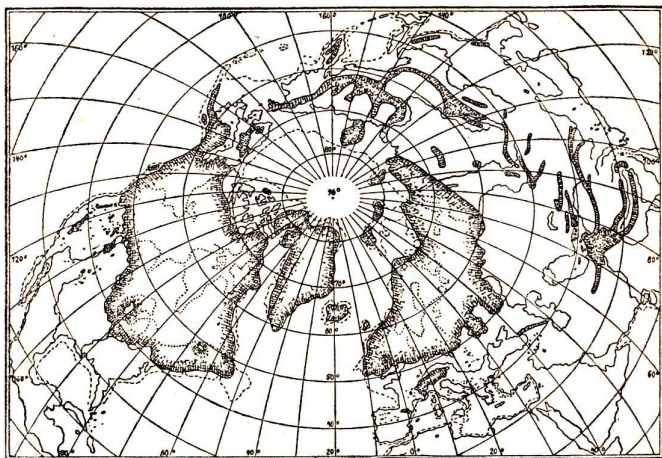
Abb. 3. Maximale Ausdehnung der diluvialen Vereisungen auf der Nördlichen Halbkugel. Nach neueren sowjetischen Forschungen war Ostsibirien stärker vereist
