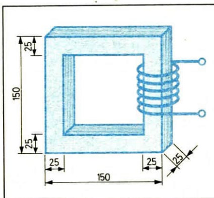
Bild 5/8 Spule mit Eisenkern
