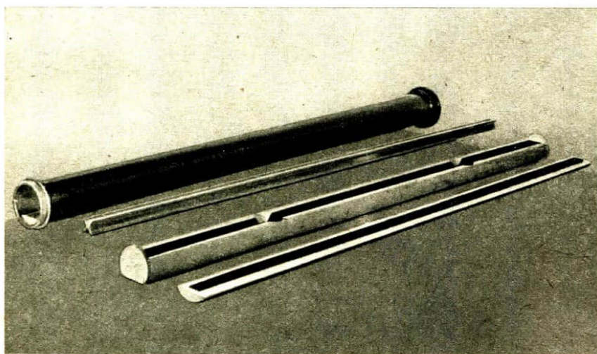
Bild 2/4 Urmeter (Gesamtansicht)
