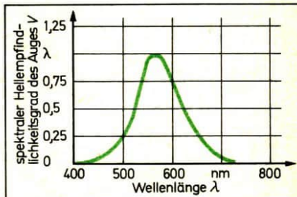
Bild 3/4 V - \lambda -Kurve
