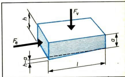
Bild 5/4 Keil mit Angabe der Bestimmungsstücke
