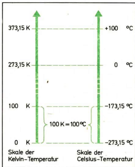
Bild 3/2 Gegenüberstellung von Kelvin- und Celsiusskale
