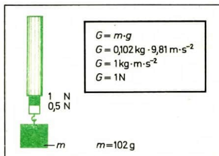
Bild 3/1 Federkraftmesser mit Teilung in Newton
