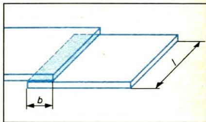
Bild 5/6 Überlappende Bleche
