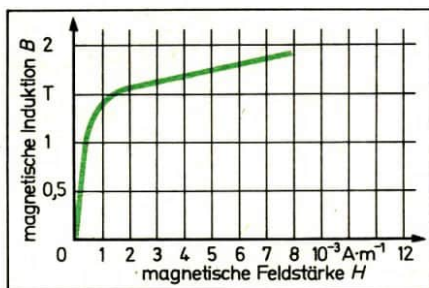
Bild 3/3 Zusammenhang zwischen magnetischer Induktion und magnetischer Feldstärke für eine bestimmte Stahlsorte
