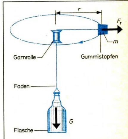
Bild 5/5 Freihandversuch zur Radialkraft
