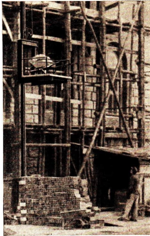
Abb. 105/1. Lastenaufzug. An einer senkrechten Führungsschiene gleitet eine nach außen geschwenkte Plattform, die die Last trägt. Hat die Plattform die gewünschte Höhe erreicht, so wird sie auf das Gerüst zum Haus hin eingeschwenkt und entladen.
