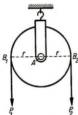
Abb. 70/1. Die feste Rolle als zweiseitiger gleich-armiger Hebel. Beide Hebelarme sind als Radien einander gleich. In den Abbildungen 70/1, 71/1, 71/2, 71/3 und 71/5 bedeutet P_1 die zu hebende Last, P_2 die dazu erforderliche Kraft.
