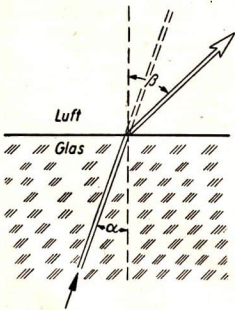
Abb. 21/2. Brechung beim Übergang des Lichts von Glas in Luft
