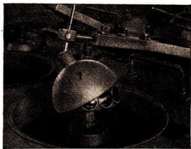
Abb. 26/4. Das Schleifen von Linsen 1 halbkugelförmige Polierschale 2 halbkugelförmiger Tragkörper
