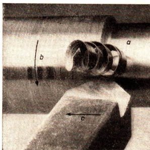
Abb. 95/3. Langdrehen mit geradem Drehmeißel.
