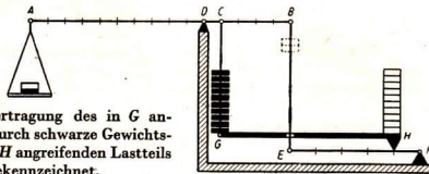
Abb. 67/1. Dezimalwaage im Gebrauch beim Abwägen eines Kartoffelsacks.
