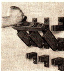
Abb. 63/5. Hebelschalter an einer Schalttafel
