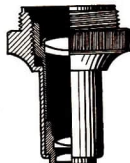
Abb. 42/2. Schnitt durch ein Mikroskopobjektiv
