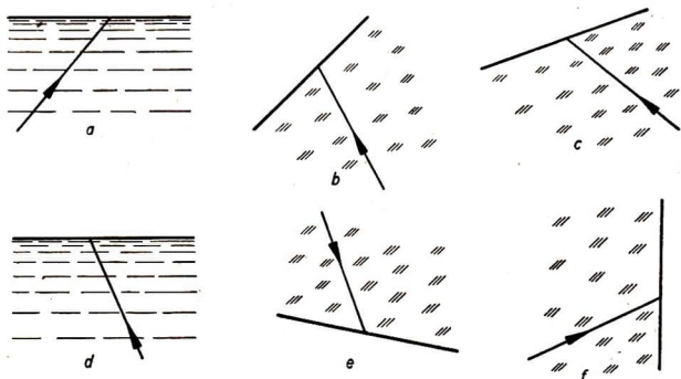
Abb. 23/2. Verschiedene Beispiele für die Brechung beim Übergang von Wasser in Luft (a und d) und von Glas in Luft (b, c, e und f)
