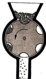
Abb. 99/2 Die Wirkungsweise der Särräder (schematisch)
