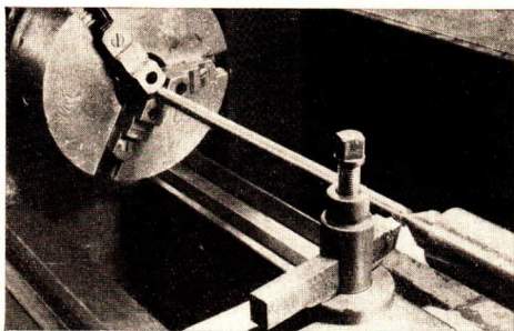
Abb. 95/1. Einspannen eines langen Werkstücks. Links ist das Spannfutter, rechts der Reitstock zu sehen.
