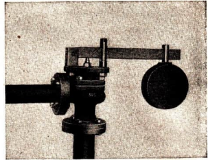
Abb. 64/1. Stange am Sicherheitsventil
