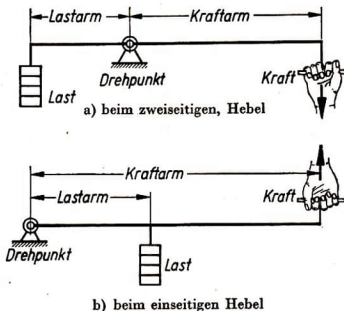
Abb. 60/2. Lage der Hebelarme
