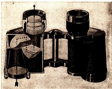
Abb. 45/1. Prismenfernglas des VEB Carl Zeiss Jena. Eine Seite ist aufgeschnitten, damit der Lichtweg sichtbar wird.
