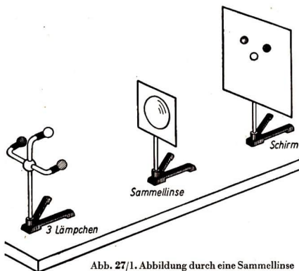
Abb. 27/1. Abbildung durch eine Sammellinse
