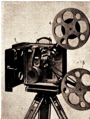
Abb. 38/1. Schmalfilmvorführgerät des VEB Carl Zeiss Jena für 16-mm-Film. Die Seitenwand ist aufgeklappt. 1 Lampengehäuse, 2 Objektiv, 3 Film, 4 Abwickelspule, 5 Aufwickelspule, 6 Ventilator
