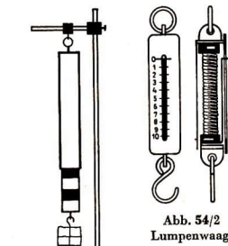
Abb. 54/1 Maeyssche Federwaage
