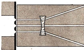
Abb. 26/2. Wirkung einer Zerstreuungslinse auf achsenparallele Strahlen
