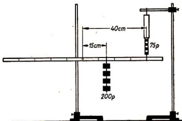
Abb. 62/1. Einseitiger Hebel Last 200 p, Lastarm 15 cm, Kraft 75 p, Kraftarm 40 cm. 200 \cdot 15 \text{ pcm} = 75 \cdot 40 \text{ pcm} .
