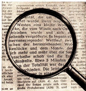
Abb. 39/1. Durchsicht durch ein Leseglas
