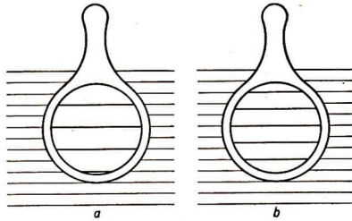
Abb. 47/1. Die Vergrößerung durch eine Lupe
