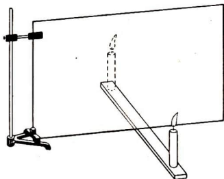
Abb. 14/1. Spiegelbild einer brennenden Kerze an einer senkrecht stehenden Glasscheibe
