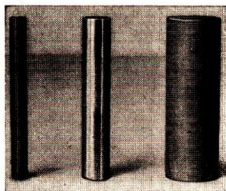
Abb. 57/1. Drei Zylinder aus Eisen, Aluminium und Holz. Sie haben gleiches Gewicht, aber verschiedenen Rauminhalt.
