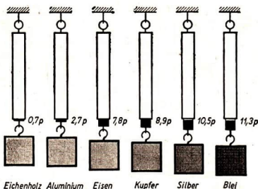
Abb. 57/2. Die Wichte verschiedener Stoffe, dargestellt durch die Gewichte von Würfeln mit einem Rauminhalt von je 1 cm 3
