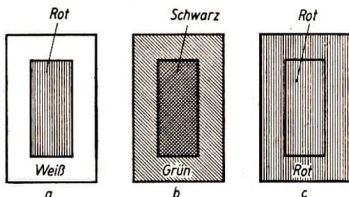
Abb. 50/1. Farbeeindruck einer roten Körperfarbe bei Bestrahlung a) mit weißem Licht, b) mit grünem Licht, c) mit rotem Licht
