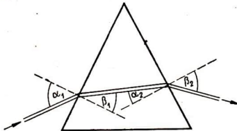
Abb. 47/3. Erklärung der Brechung durch ein Glasprisma nach dem Brechungsgesetz
