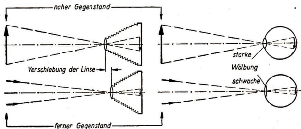
Abb. 34/2. Vergleich der Abbildung eines entfernten und eines nahen Gegenstandes im Auge und in der Kamera
