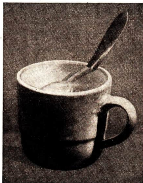
Abb. 19/2. Ein in einer Tasse mit Wasser stehender Löffel erscheint an der Wasseroberfläche geknickt.
