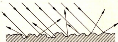
Abb. 16/2. Diffuse Reflexion des Lichts an einer rauen Fläche.
