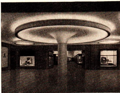
Abb. 16/2. Diffuse Reflexion des Lichts an einer rauen Fläche.
