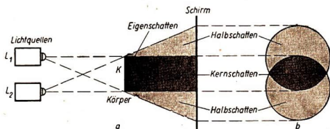
Abb. 9/2 Entstehen des Schattens bei Beleuchtung durch zwei Lichtquellen
