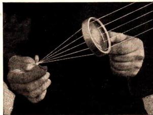
Abb. 25/2. Entzünden eines Streichholzes mit Hilfe einer Sammellinse. Die im Bild sichtbaren Lichtstrahlen sind nachträglich eingezeichnet.
