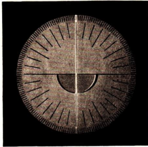
Abb. 21/1. Verlauf eines Lichtstrahles bei senkrechtem Auffall auf eine Glasfläche
