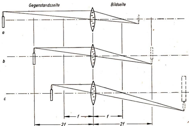
Abb. 28/1. Drei Fälle der reellen Abbildung
