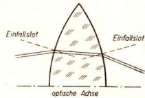
Abb. 25/1. Die Brechung eines Lichtstrahls an einer Sammellinse
