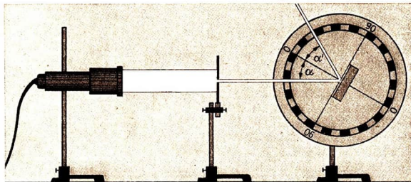
Abb. 13/1. Vergleich von Einfallswinkel und Reflexionswinkel an einer optischen Scheibe
