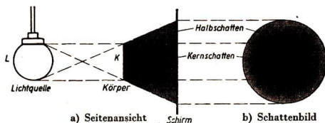
Abb. 9/3 Kernschatten und Halbschatten bei Beleuchtung eines Körpers durch eine ausgedehnte Lichtquelle. Der Halbschatten nimmt nach außen hin an Helligkeit zu.
