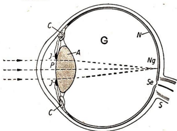
Abb. 34/1. Waagerechter Schnitt durch das Auge (schematisch). I Iris (Regenbogenhaut); P Pupille, Sechloch in der Regenbogenhaut; N Netzhaut, sie ist die lichtempfindliche Schicht des Auges und enthält die Enden der Sehnervfasern; Ng Netzhautgrube; S Sehnerv; Se Sehnervende; A Augenlinse, durchsichtig, elastisch, in der Wölbung veränderlich; C Ziliarmuskel, Muskel zum Verändern der Linsenkrümmung; G Glaskörper, aus einer gallertartigen, durchsichtigen Masse bestehend
