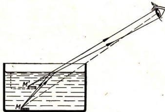
Abb. 21/3. Verlauf der Lichtstrahlen beim scheinbaren Heben eines Gegenstandes im Wasser
