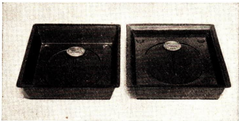
Abb. 19/1. Scheinbare Hebung einer Münze. Links: Münze in leerer Schale. Rechts: Schale mit Wasser gefüllt. Der Boden mit der Münze scheint gehoben zu sein.
