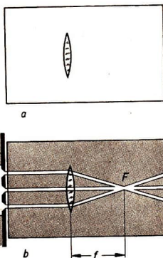
Abb. 24/1. Der Strahlengang an einer Sammellinse
