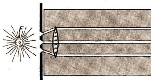
Abb. 26/1. Erzeugung achsenparalleler Lichtstrahlen mit Hilfe einer Sammellinse
