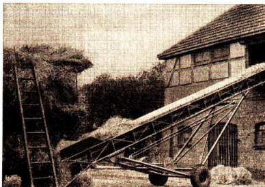
Abb. 81/2. Transportband zum Befördern von Stroh in einen Speicher
