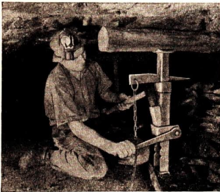
Abb. 89/3. Bergmann beim Festkeilen einer Deckenstütze in einer Kupferschiefgrube des volkseigenen Mansfelder Bergbaus.
