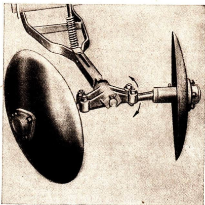
Abb. 87/1. Zudeck-Scheiben an der Kartoffellegemaschine
