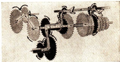
Abb. 100/1. Vielstufengetriebe einer Drillmaschine
