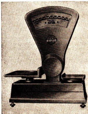
Abb. 66/3. Zeiger-Schnellwaage
