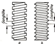
Abb. 83/1 Die häufigsten Gewindeformen
