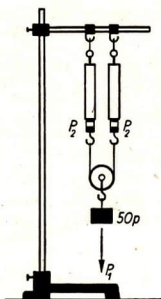
Abb. 71/2 Zwischen zwei Feder- waagen hängende lose Rolle. Jede Federwaage nimmt die Hälfte der Last auf. P_2 = \frac{P_1}{2} .
