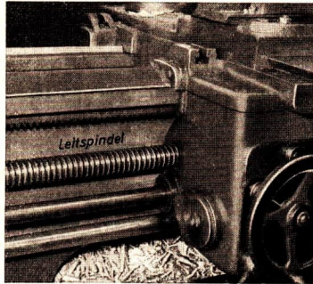
Abb. 85/1. Leitspindel einer Drehmaschine
