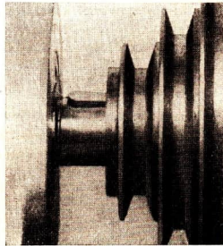
Abb. 89/4 Verbindungskeil
