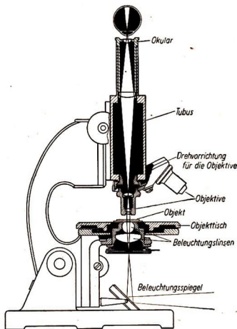
Abb. 42/1. Achsenschnitt durch ein Geradsicht-Mikroskop mit eingezeichnetem Strahlengang
