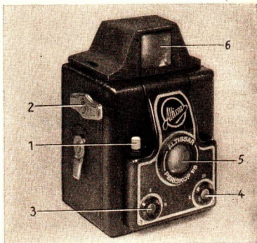
Abb. 32/1. Rollfilm-Boxkamera „Altissa“, hergestellt vom VEB Altissa-Camera-Werk, Dresden. 1 Auslöseknopf, 2 Kurbel für Filmtransport, 3 Einstellung der Blende, 4 Einstellung der Verschlusszeiten, 5 Objektiv, 6 Durchblicksucher
