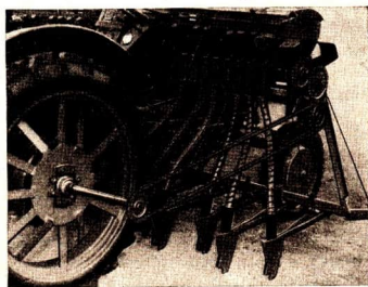
Abb. 100/2. Die Saatleiter einer Drillmaschine, darunter die Drillschare
