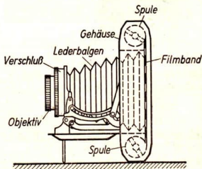
Abb. 32/3 Schnitt durch eine Rollfilm-Klappkamera
