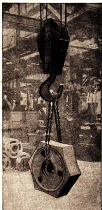
Abb. 71/4. Unterer Block eines großen Flaschenzuges mit Traghaken und angehängter Last
