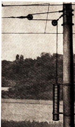
Abb. 72/2. Einfacher Flaschenzug als Halte- und Spannvorrichtung für den Fahrdrabt einer Straßenbahn. Verwendet wird eine lose, eine feste Rolle und an Stelle des Seiles eine Kette. Sie wird durch schwere Betonscheiben gespannt. Die auf den Fahrdrabt ausgeübte Zugkraft ist doppelt so groß wie das Gewicht der Betonscheiben.
