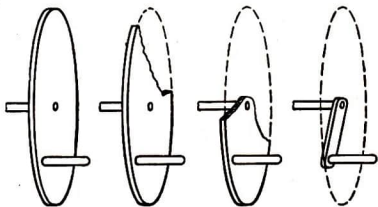
Abb. 74/1. Entwicklung einer Kurbel aus einem Wellrad.
