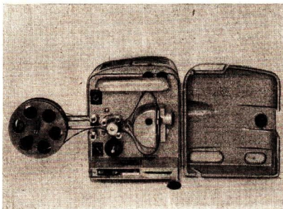
Abb. 38/1. Schmalfilmvorführgerät des VEB Carl Zeiss Jena für 16-mm-Film. Die Seitenwand ist aufgeklappt. 1 Lampengehäuse, 2 Objektiv, 3 Film, 4 Abwickelspule, 5 Aufwickelspule, 6 Ventilator
