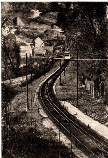
Abb. 69/1. Drahtseilbahn zum Weißen Hirsch in Dresden-Loschwitz. Durch Drahtseile, die zwischen den Schienen über Rollen laufen, werden die Wagen gezogen.
