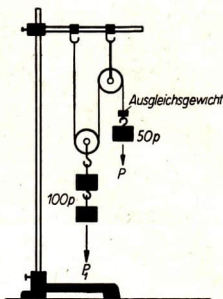
Abb. 71/3 Verbindung einer losen und einer festen Rolle. Die Gegen- kraft ist halb so groß wie die an der losen Rolle angreifende Last. P_2 = \frac{P_1}{2} .
