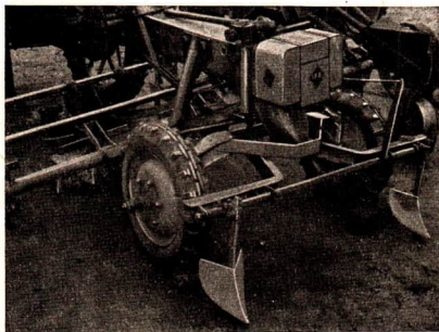
Abb. 86/2. Häufelkörper vor den Vorderrädern eines Traktors
