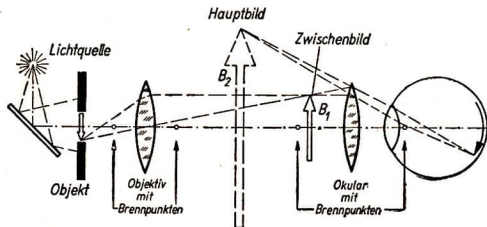
Abb. 41/2. Versuchsanordnung zur Veranschaulichung der Wirkungsweise eines Mikroskops
