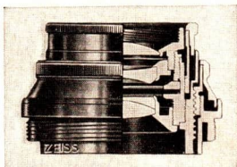
Abb. 30/1. Objektiv Zeiss-Tessar
