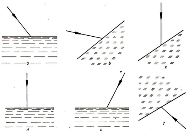
Abb. 23/1. Verschiedene Beispiele für die Brechung beim Übergang von Luft in Wasser (a, d und e) sowie von Luft in Glas (b, c und f)
