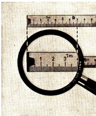
Abb. 40/1. Betrachten eines Gliedermaßstabes ohne Lupe (oben) und mit Lupe (unten). Es ergibt sich ein Vergrößerungsmaßstab von rund 1,75 : 1.
