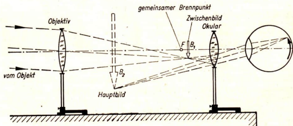
Abb. 44/2. Die Wirkungsweise des astronomischen Fernrohrs. Der weit entfernte Gegenstand (Stern) wird vom Objektiv in B_1 abgebildet. Das reelle Bild wird durch das Okular vergrößert betrachtet (vgl. Lupenwirkung Abb. 41/1).
