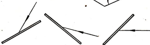
Abb. 17/2. Spiegel und einfallender Strahl in verschiedenen Richtungen
