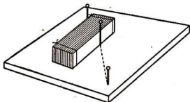
Abb. 22/1. Stecknadelversuch zur Brechung. Die drei Nadeln werden durch den Glasplattensatz hindurch in eine Visierlinie gebracht
