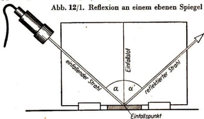
Abb. 12/1. Reflexion an einem ebenen Spiegel
