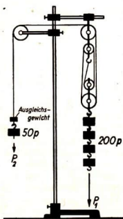
Abb. 71/5 Modell eines aus zwei losen und zwei festen Rollen bestehenden Flaschenzuges. Die Rollen sind am Modell der besseren Erkennbarkeit halber übereinander ange- ordnet. Bei der technischen Ausführung liegen sie stets nebeneinander.
