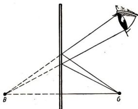
Abb. 14/3. Vom Gegenstandspunkt G gehen Strahlen aus, werden am Spiegel reflektiert und treffen in unser Auge. Sie scheinen vom Bildpunkt B herzukommen.
