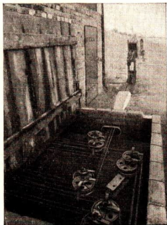
Abb. 69/2. Umlenkrollen im Rollenkasten eines mechanischen Stellwerkes der Eisenbahn.
