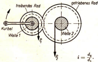
Abb. 75/3. Schema einer Zahnradübertragung. In schematischen Zeichnungen werden Zahnräder durch einen Vollkreis mit eingezeichnetem gestricheltem Kreis wiedergegeben. Das auf der Kurbelwelle (Welle 1) sitzende Zahnrad (treibendes Rad) greift in ein größeres Zahnrad (getriebenes Rad) ein, das mit der Welle 2 verbunden ist.
