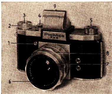
Abb. 33/1. Kleinbildkamera „Praktica“, hergestellt von den volkseigenen Kamerawerken Niedersieditz, Dresden. Zeiss-Objektiv Tessar, Brennweite 50 mm, Bildgröße 24 mm \times 36 mm. Die Sucheröffnung ist aufgeklappt. 1 Auslöseknopf, 2 Filmtransportknopf, 3 Bildzählscheibe, 4 Einstellknopf für Verschlusszeiten, 5 Rückspulknopf, 6 Objektiv, 7 Einstellung für die Blendenöffnung, 8 Einstellung für die Entfernung, 9 Sucher
