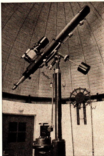
Abb. 44/1. Astronomisches Fernrohr in der Schulsternwarte der Pestalozzi-Schule in Rode- wisch im Vogtland. Das Rohr trägt seitlich eine photographische Kamera für Sternaufnahmen, einen Astrographen.
