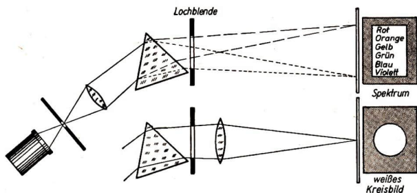
Abb. 49/1. Versuchsanordnung zur Wiedervereinigung der Spektralfarben zu Weiß. Der Schirm ist in die Zeichenebene geklappt.
