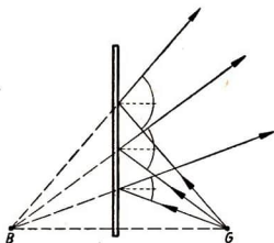
Abb. 14/2 Reflexion von Lichtstrahlen am ebenen Spiegel. Die Strahlen gehen von einem Punkt aus.
