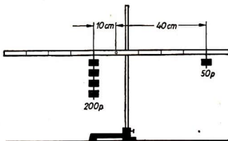
Abb. 61/1. Zweiseitiger Hebel. Last 200 p, Lastarm 10 cm, Kraft 50 p, Kraftarm 40 cm
