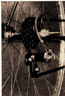
Abb. 92/1. Gangschaltung (Vier Zahnkränze)
