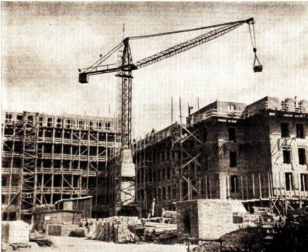
Abb. 77/2. Turmdrehkran
