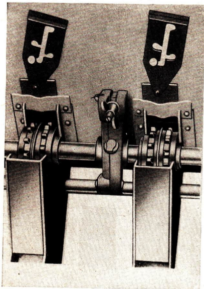
Abb. 99/1. Die Särräder einer Drillmaschine
