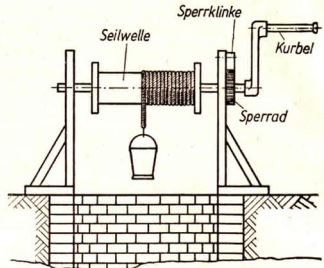
Abb. 75/2. Einfache Seilwinde als Hebevorrichtung über einem offenen Brunnen.
