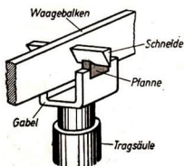
Abb. 65/1. Schneidenaufhängung des Waagebalkens. Durch den Waagebalken ragt eine keilförmige Schneide. Sie ruht auf zwei Pfannen, die mit dem Gestell fest verbunden sind.
