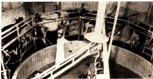
Abb. 42 Moderne Melkanlage in der Forschungsstelle für Landarbeit Gundorf. Wie bei einem Fischgräten-Melkstand, so kann auch bei dieser Anlage ein Melker stündlich 50 Kühe melken.
