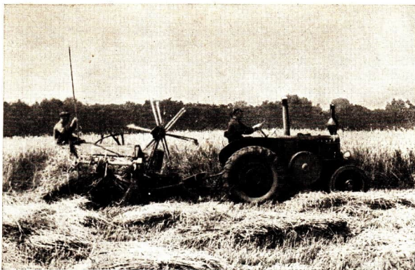
Abb. 36 Mähbinder bei der Arbeit
