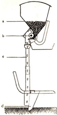
Abb. 34 Drillmaschine. Das Saatgut im Saatkasten (a) fällt beim Drehen des Zahnrädchens (b) in das Särohr (c). Die Schar (d) reißt den Boden auf, in den die Körner fallen.
