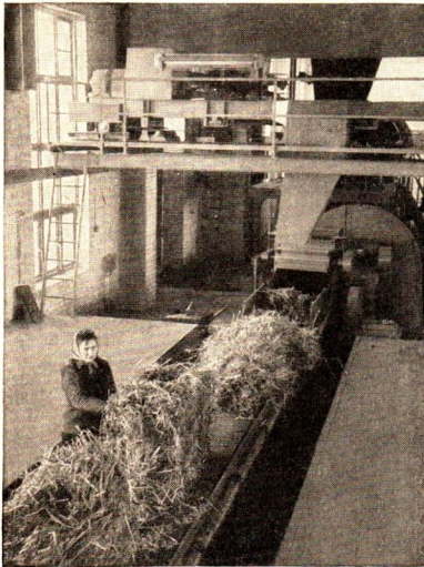
Abb. 18 Herstellung von Preßplatten aus Stroh im Faserplattenwerk. Transportbänder bringen das Stroh in die Maschine.
