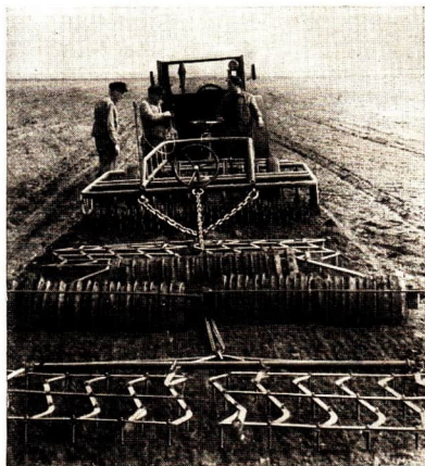
Abb. 40 Traktoristen der MTS Cröbern bestellen ein 10 ha großes Feld der LPG in Holzhausen. Viele Geräte sind miteinander gekoppelt.
