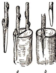
Abb. 145. Zwei Arten des Pfropfens
