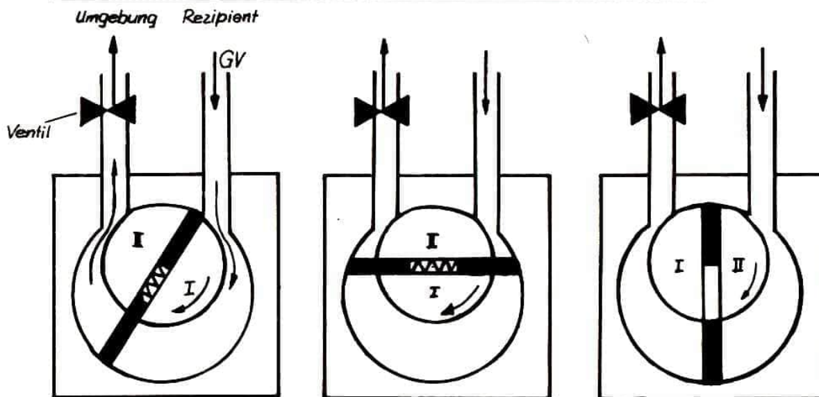
Abb. 1 Prinzip einer einstufigen Drehschieberpumpe
