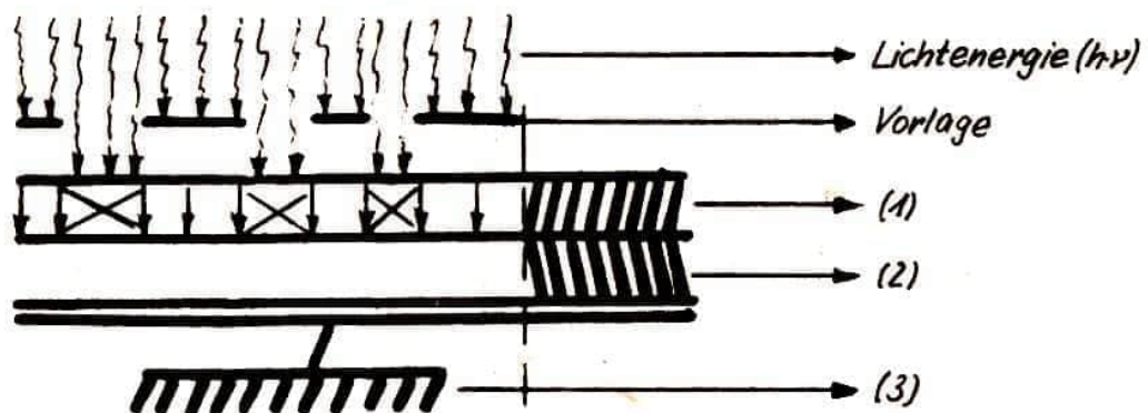
Abb. 3 Darstellung des Feldlinienverlaufes ( \downarrow ) beim Belichten (x - an diesen Stellen fließen die Ladungen beim Belichten ab)
