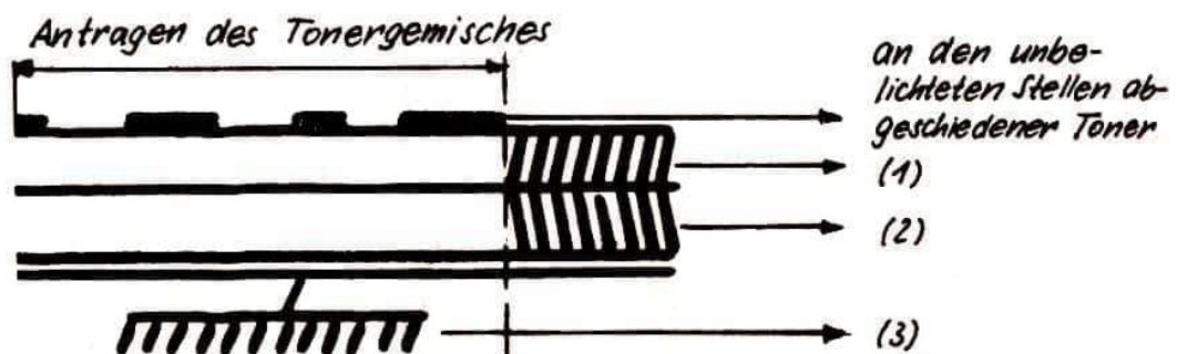
Abb. 4 Entwicklung des latenten elektrischen Bildes
