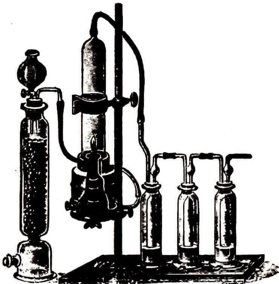
Schwefelbestimmungsapparat nach Drehschmidt
