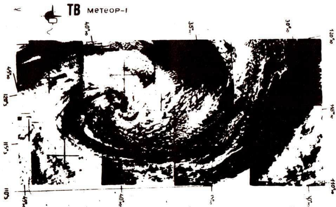
Aufnahme eines Tiefdruckwirbels durch den sowjetischen Wettersatelliten METEOR - 1 am 15. 4. 69
