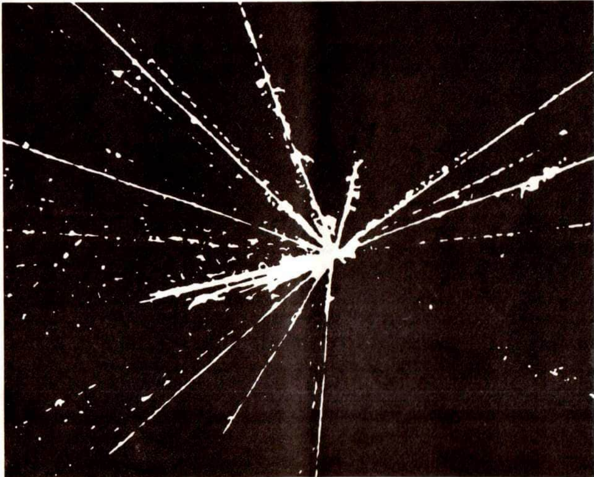
Kernzerfall
