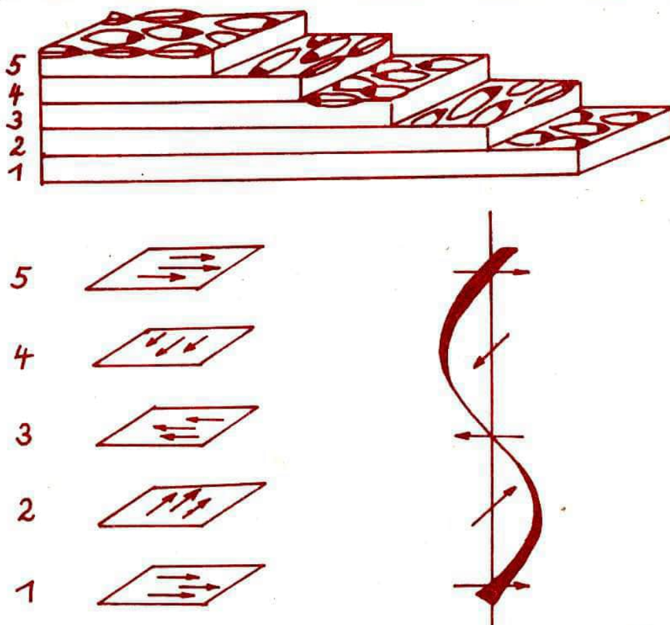
Abb. 3 Die Struktur einer cholesterinischen Phase
