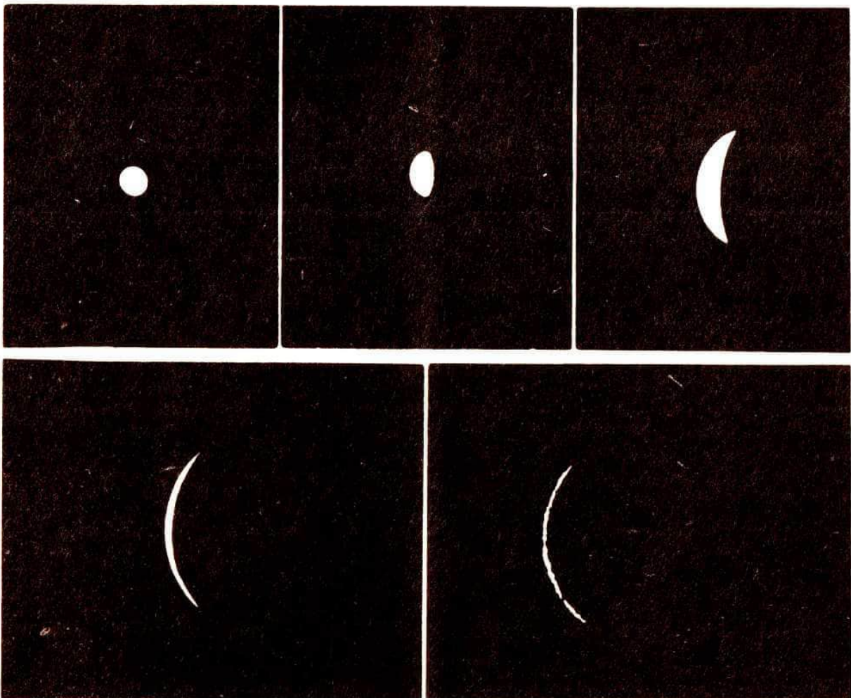
Phasenänderung der Venus bei einem Umlauf um die Sonne, von der Erde aus gesehen. Links oben obere, rechts unten untere Konjunktion. Die Vergrößerung ist bei allen fünf Aufnahmen konstant.
