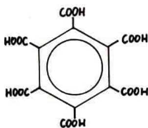
Mellitsäure
