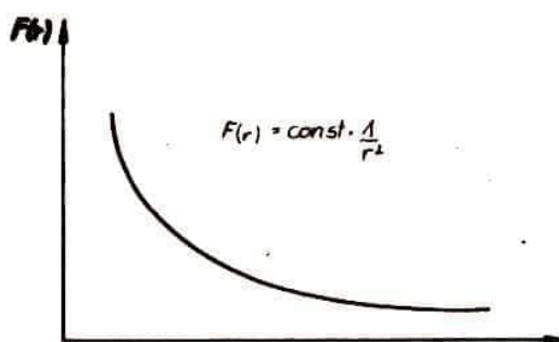
Abhängigkeit der Schwerkraft K von der Entfernung
