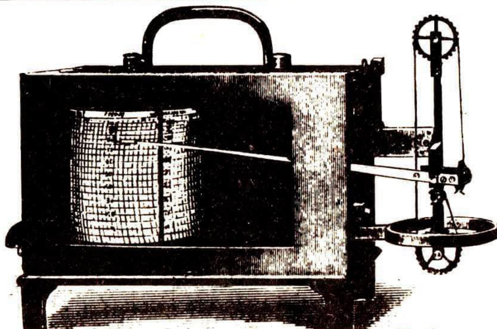
Selbstregistrierender Luftfeuchtigkeits-Meßer von Fuchs
