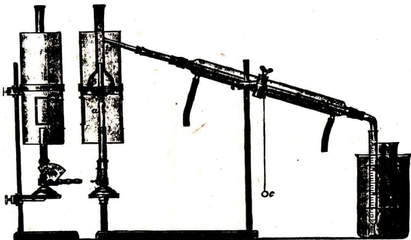
Destillationsapparat für Benzin
