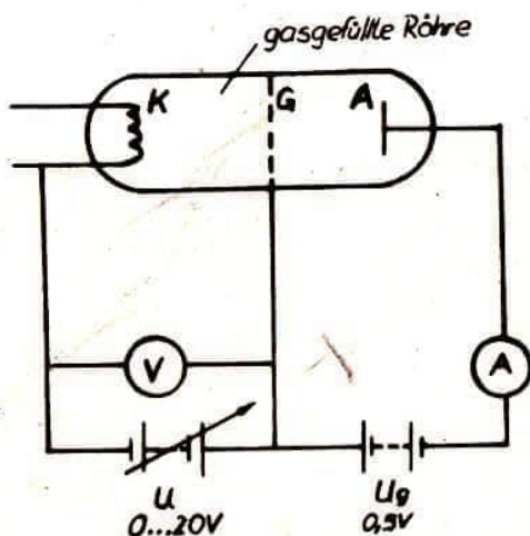
Abb. 1 Aufbau des Franck - Hertz - Versuches
