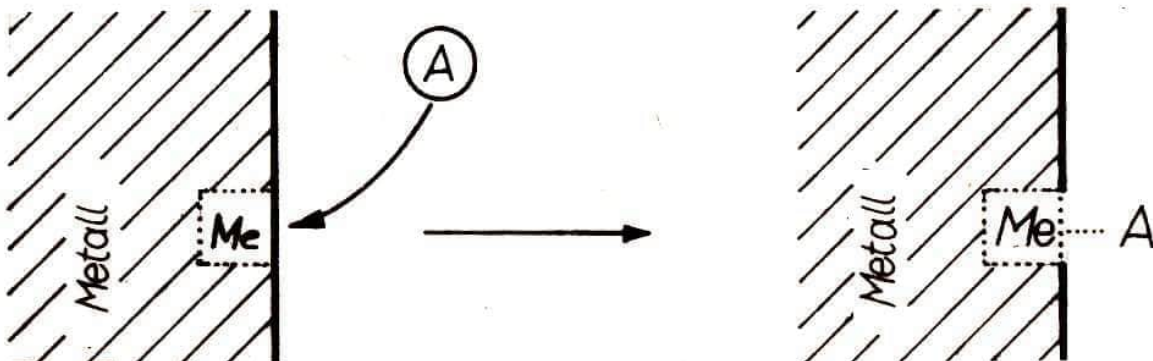
Abb. 2 Bildung einer Oberflächenverbindung
