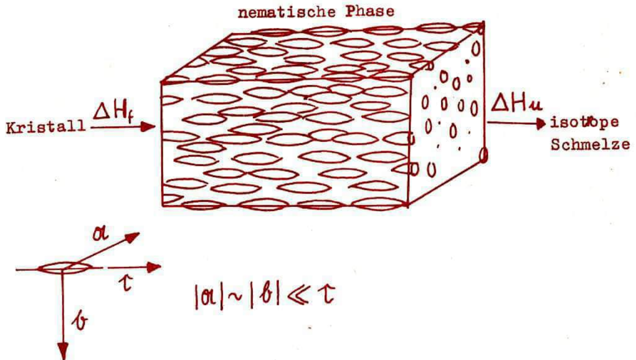
Abb. 2 Entstehung einer nematischen Phase
