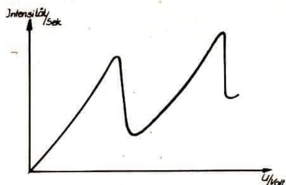
Abb. 2 Beispiel für ein U - I - Diagramm bei Quecksilberdampfzuführung
