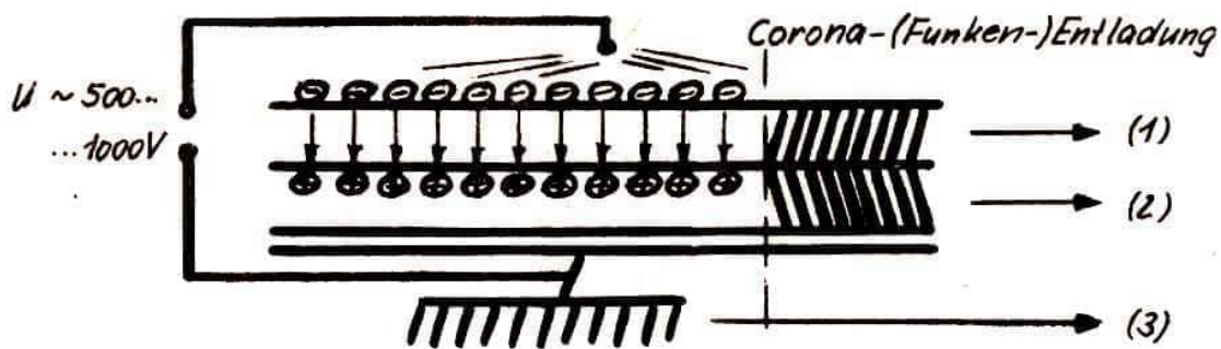
Abb. 2 Darstellung der Ladungsverteilung und des Feldlinienverlaufes ( \downarrow ) während der Aufladung
