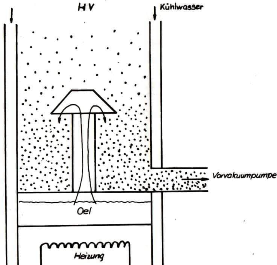
Abb. 2 Prinzip einer Öldiffusionspumpe
