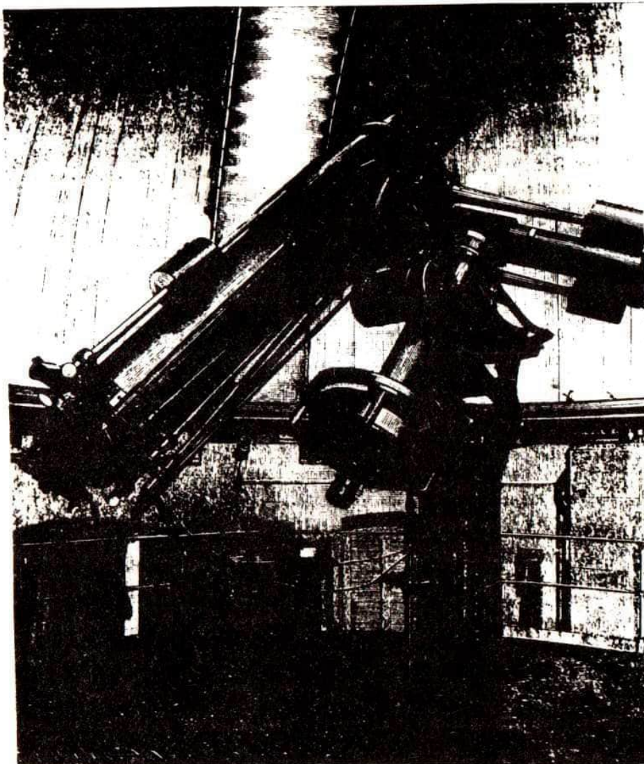
Äußere Ansicht eines großen beweglichen Refraktors nach den Bedürfnissen der modernen Astronomie.
