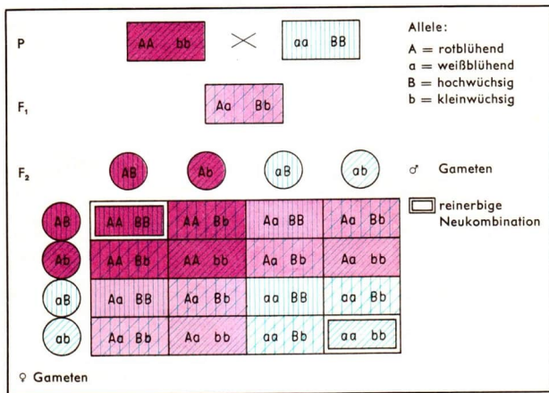
Kreuzungsschema
