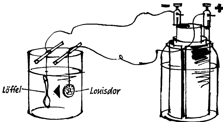
Galvanische Vergoldung
