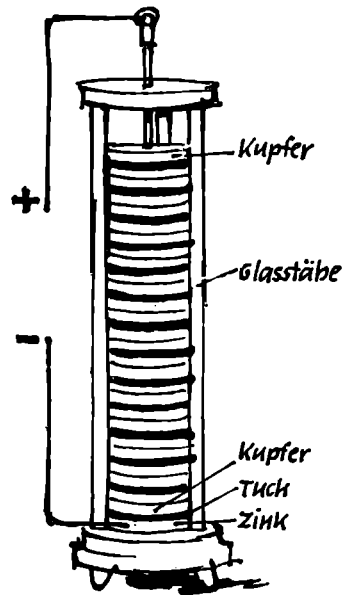
Voltasäule
