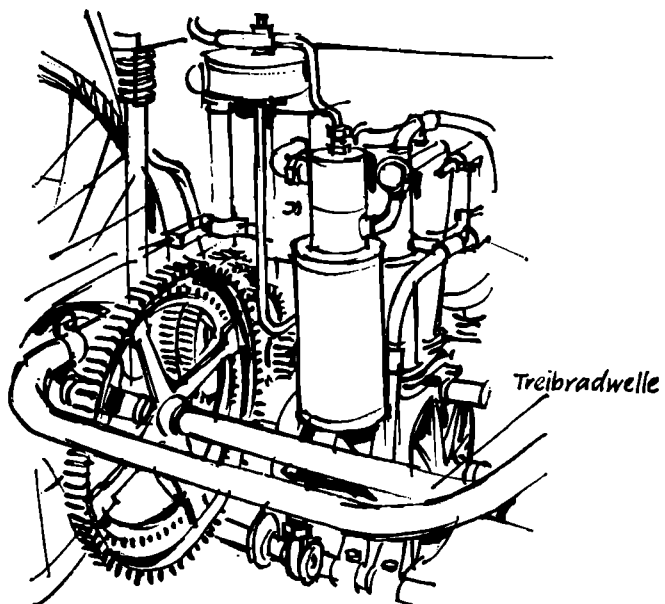
Antrieb des Daimler-Stahl- radwagens von 1889
