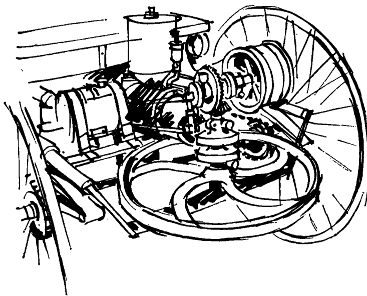
Benz' dreirädriger Motor- Wagen (Motor, Kupplung und Getriebe)
