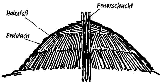
Holzkohlenmeller (Schnitt)
