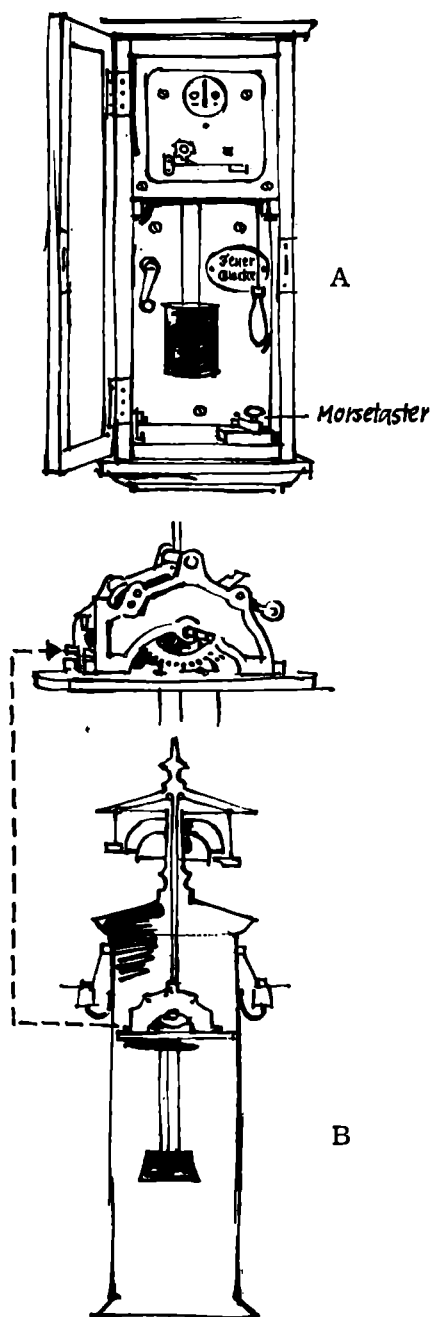
A Feuermelder B Läutewerk
