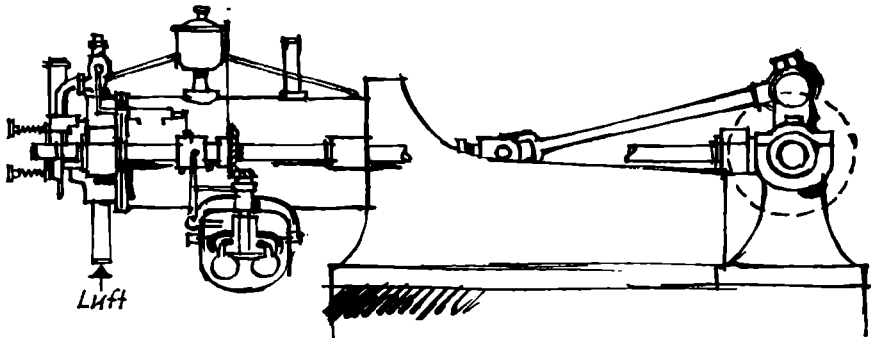
Viertaktmotor, mitgestaltet von Daimler (Schnitt)
