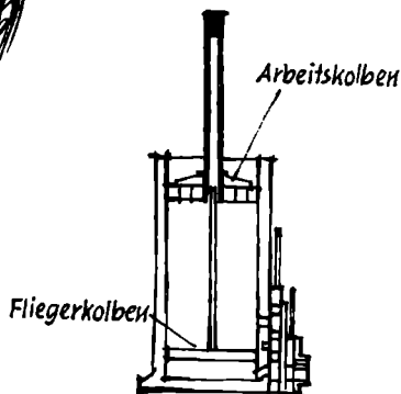
Ottos Gasmotor mit Schema
