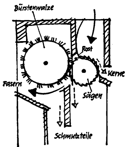
Cotton-Gin (Schnlitt)
