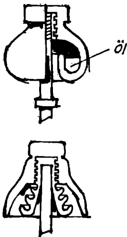
Ölisolatoren
