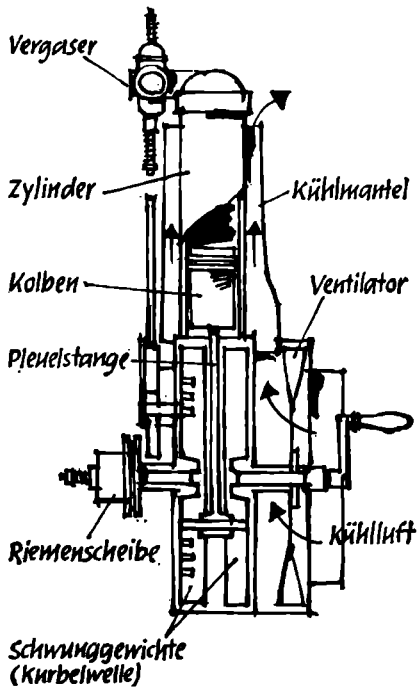
Daimlers erster Fahrzeugmotor (Schnitt)
