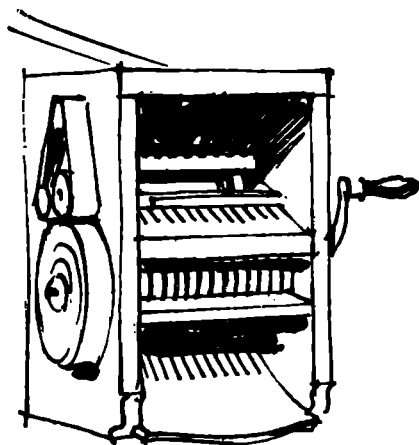
Cotton-Gin, Whitneys neues Modell
