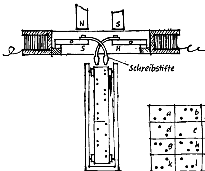
Steinhells Telegraf
