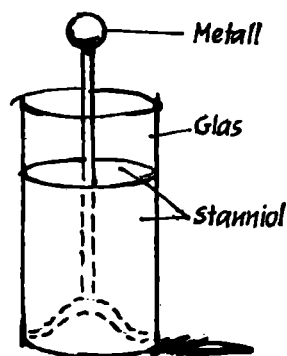
Kleistsche oder Leidener Flasche
