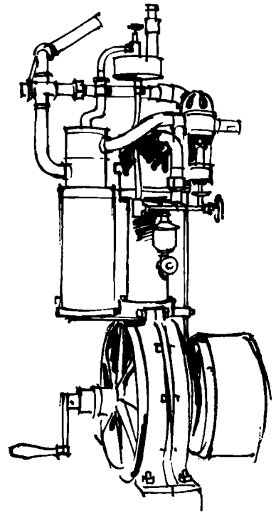
Daimlers Einzylindermotor, 1885
