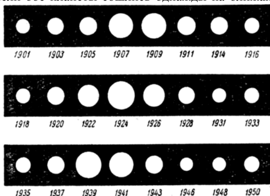
Рис. 65. Изменение видимого диаметра Марса в различные противостояния XX в. В 1909, 1924 и 1939 гг. были великие противостояния.
