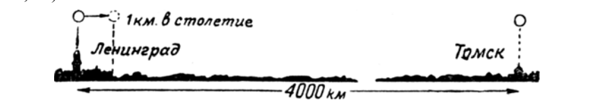
Рис. 83. Масштаб звёздных движений. Два крокетных шара, один в Ленинграде, другой в Томске, движутся со скоростью 1 км в столетие — вот уменьшенное подобие сближения двух звёзд. Из этого ясно, как ничтожна вероятность столкновений между звёздами.
