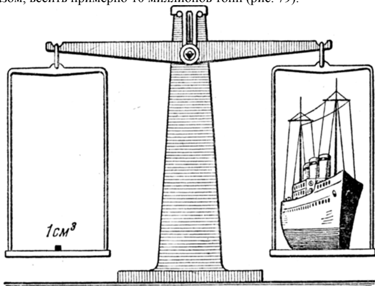
Рис. 79. Один кубический сантиметр атомных ядер мог бы уравновесить океанский пароход даже и при весьма неплотной упаковке их. Плотнo же уложенные в объёме 1 \text{ см}^3 атомные ядра весили бы 10 миллионов тонн!
