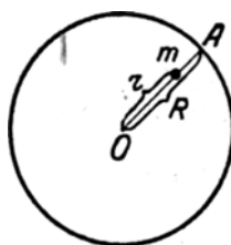
Рис. 97. К вычислению изменения веса тела с приближением к центру планеты.
