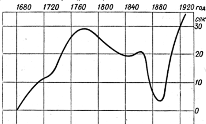
Рис. 29. Эта кривая показывает, как с 1680 по 1920 г. вращение Земли отклонялось от равномерного вращения. Если бы Земля вращалась равномерно, то на графике это изобразилось бы горизонтальной прямой. Подъёмы кривой соответствуют удлинению суток, т. е. замедлению вращения Земли; понижения — ускорению вращения.
