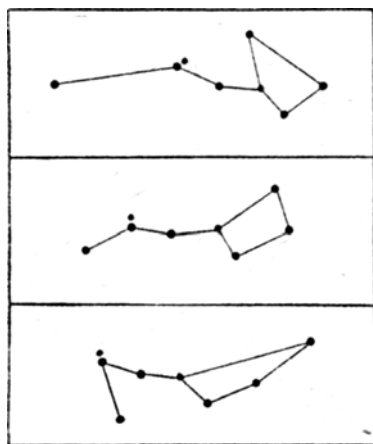
Рис. 80. Фигуры созвездий медленно меняются с течением времени. Средний рисунок изображает «ковш» Большой Медведицы в настоящее время, верхний — 100 тыс. лет назад, нижний — через 100 тыс. лет после нашего времени.
