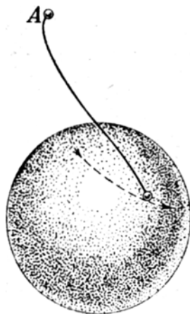
Рис. 25. Тот же путь представляется лунному наблюдателю искривлённым.
