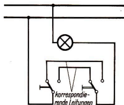
58/3 Wechselschaltung
