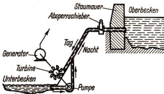
42/1 Schematische Darstellung eines Pumpspeicherwerkes
