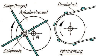
12/3 Kurvensteuerung bei einer Aufnahmetrommel
