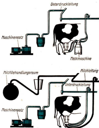
30/1 a) Kannenmelkanlage; b) Rohrmelkanlage
