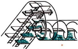
17/2 Schacht des Ährelevators und obere Ährenschncke
