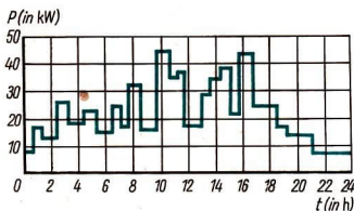
45/1 Tagesbelastungskurve eines VEG
