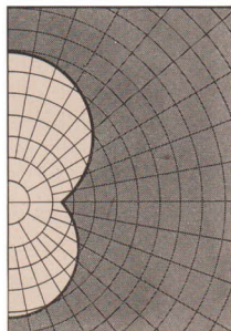
64/3 Leuchte für vorwiegend indirektes Licht; Lichtverteilung (schematisch)
