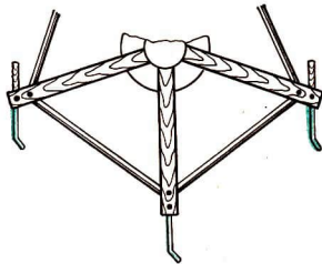
11/3 Stellung der Haspelzinken bei lagerndem und stehendem Getreide
