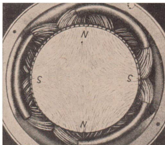
99/2 Magnetfluß einer 4-poligen Maschine
