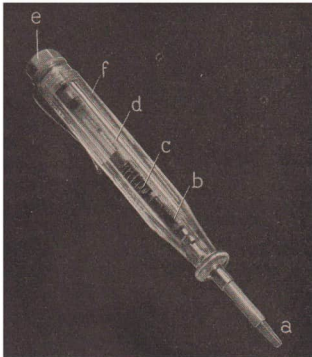
83/1 Polsucher
