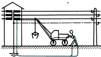
72/1 Stromkreis an einem Kran, dessen Ausleger mit der Freileitung in Verbindung steht
