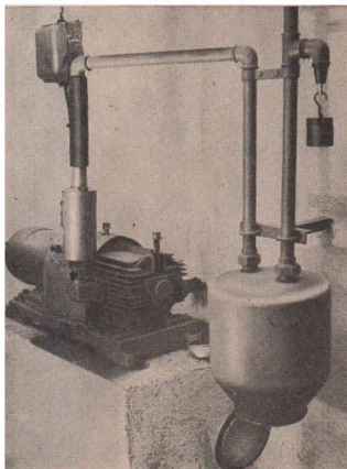
29/1 Funktionsschema und Ansicht des Maschinensatzes „Gigant“
