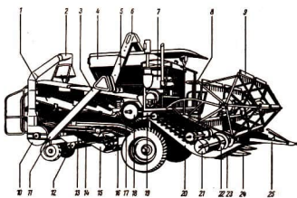
7/4 Schnittdarstellung des Mähdreschers
