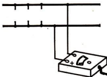
92/3 Messen des Isolationswiderstandes Leitung gegen Leitung
