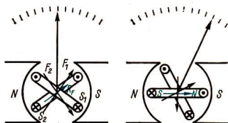
89/3 Schematische Darstellung der Wirkungsweise eines Kreuzspulmeßgerätes
