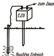
79/2 Erdung des Elektroweidezaungerätes
