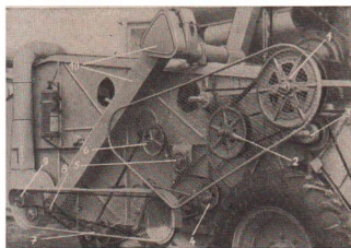
8/1 Antrieb des Mähdreschers vom Motor ausgehend
