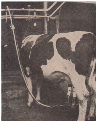
33/1 Impulsa-Rohrmelkanlage für Anbindeställe nach der Montage
