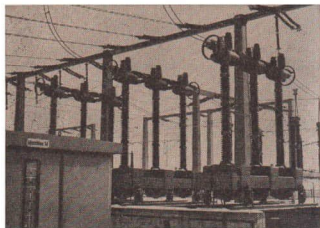
43/1 Freiluftumspannstation
