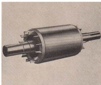
97/4 Käfigläufer
