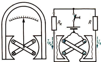
89/2 Schaltung des Kreuzspulmeßgerätes
