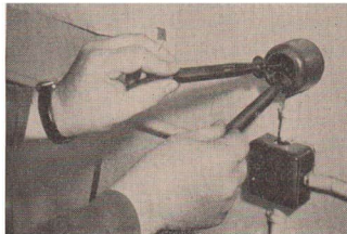
83/3 Spannungssucher
