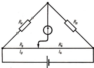
90/2 Schaltung der Schleifdrahtmeßbrücke
