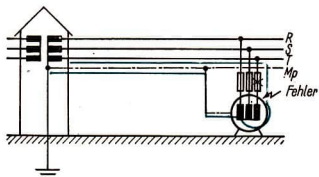
73/1 Schutzmaßnahme — Nullung
