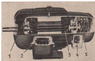
103/1 Schnittmodell eines Schleifringläufermotors
