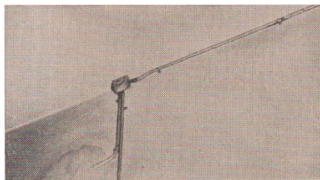
49/6 Normen-Rohrdraht-Aderleitung im Haushalt verlegt
