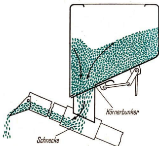
18/1 Kornbunker mit Klappe und Entleerungsschnecke
