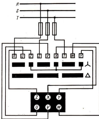
102/2 Stern-Dreieck-Schalter am Klemmbrett angeschlossen
