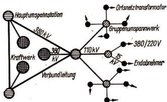
43/2 Schema der Energieverteilung
