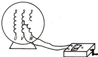
85/3 Prüfen der Wicklungen eines Drehstrommotors auf Wicklungsschluß mit Kurbelinduktor
