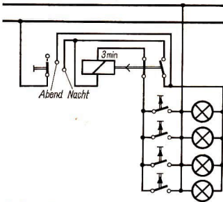
59/2 Treppenhausschaltung mit Automat
