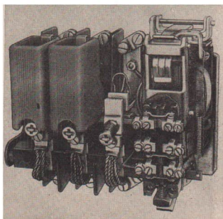
108/3 Luftschütz LF 25
