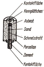
56/5 und 6 Schaltzeichen und Aufbau eines Schmelzeinsatzes
