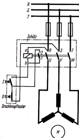
108/2 Schützschaltung für Drehstromkurzschlußläufermotor
