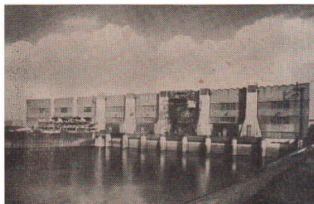
41/3 Wasserkraftwerk
