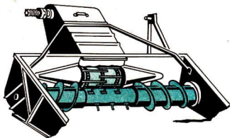
12/2 Förderschnecke und Schrägförderband
