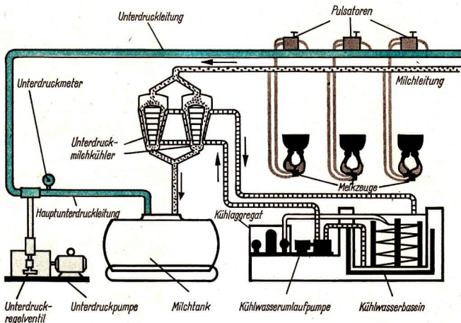
34/1 Schema der Rohrmelkanlage
