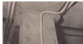
49/4 Leichtes Stahlrohr an einer Stahlkonstruktion verlegt
