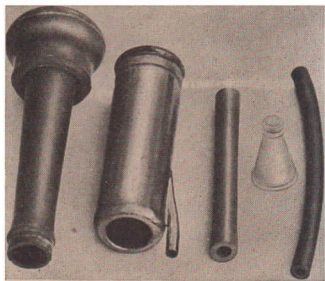
31/2 Melkbecher der Impuls-Melkmaschine
