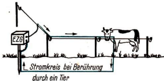
77/1 Schema einer Elektrozaunanlage
