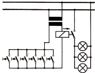
59/3 Der am Relais gezeichnete Pfeil deutet an: Das Schaltstück führt eine Drehbewegung aus
