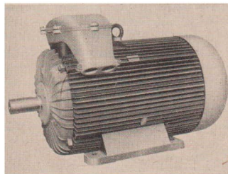
94/2 Moderner Drehstrom-Asynchronmotor
