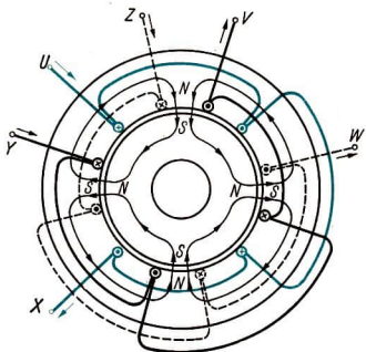
97/2 Wicklung eines Motors mit 2 Polpaaren
