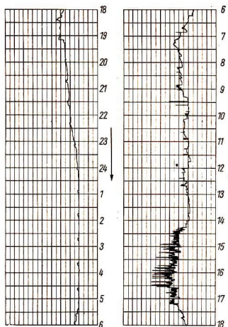
86/3 Leistungsdiagramm
