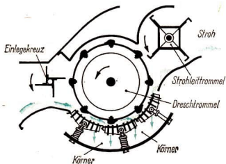
12/4 Dreschelemente
