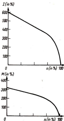
100/1 Anlaufkurven eines Drehstrom-Kurzschlußläufermotors
