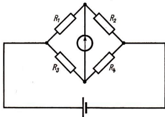
90/1 Brückenschaltung
