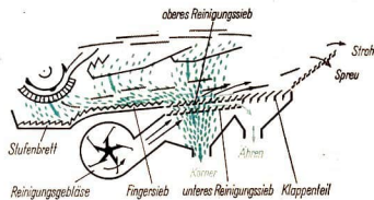
Zu ihnen gehören: Das Stufenbrett und das Fingersieb, das obere Reinigungssieb mit der Siebverlängerung und dem Kurzstrohsieb, das untere Reinigungssieb und das Gebläse.
