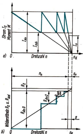
104/1 Verlauf des Stromes I_2 und des Moments M (Bild a) beim Anlassen eines Schleifringläufermotors mit Stufenwiderständen R_{An3} \dots R_{An1} (Bild b)
