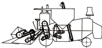
9/1 Ketten- und Riementriebe am Mähdrescher a) linke Seite; b) rechte Seite
