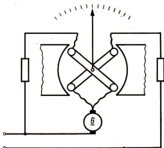
92/2 Prinzipschaltung eines Kurbelinduktors
