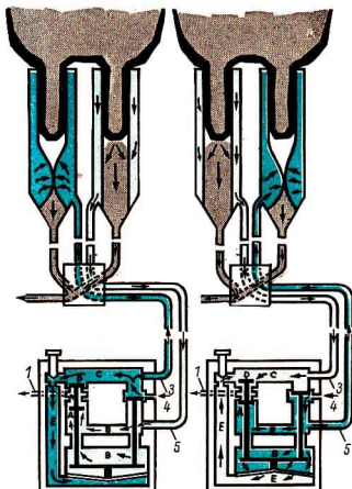
32/2a Saugtakt durch den Membranpulsator
