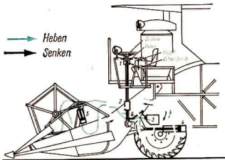
11/1 Funktion der Hubzylinder am Schneidwerk und an der Haspel
