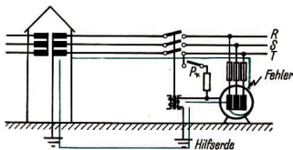
73/2 Fehlerspannungsschutzschalter
