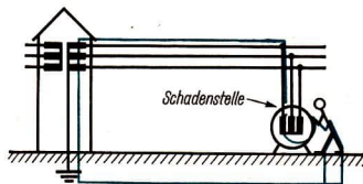
72/2 Stromkreis an einem Körperschluß aufweisenden Motor
