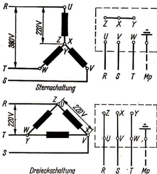
101/1 Stern- und Dreieckschaltung
