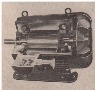
97/1 Kurzschlußläufermotor, Schnittmodell
