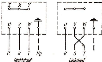
102/1 Ändern der Drehrichtung
