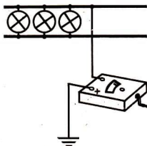
92/4 Messen des Isolationswiderstandes einer ganzen Anlage oder eines Teilstückes gegen Erde
