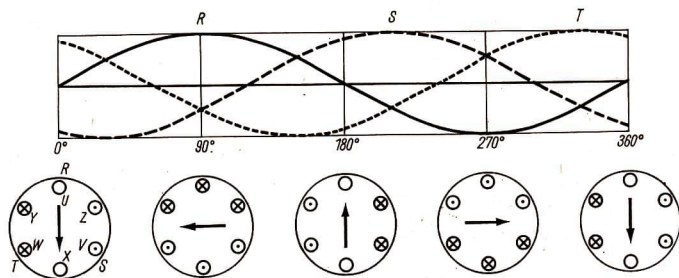
98/1 Entstehung des Drehfeldes bei einer 2-poligen Maschine
