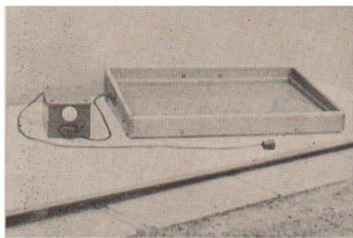
69/1 Elektrisch beheiztes Ferkelnest mit Schutztransformator
