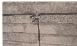
49/8 NYIF-Leitung auf dem Mauerwerk, geheftet
