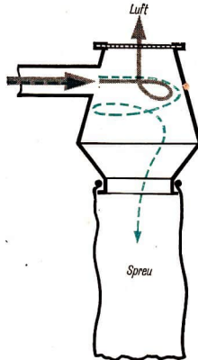
17/3 Spreuzyklon
