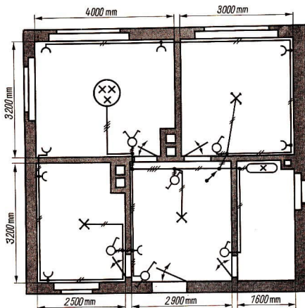
48/1 Installationsplan einer Wohnung
