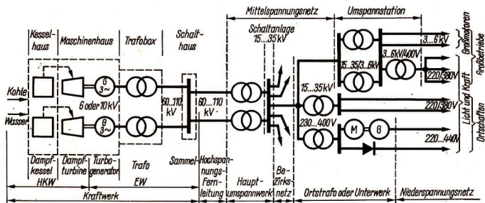
47/1 Schema des Energieflusses vom Kraftwerk zum Abnehmer
