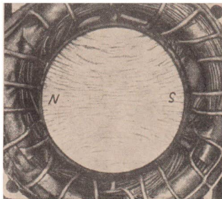
99/1 Magnetfluß einer 2-poligen Maschine
