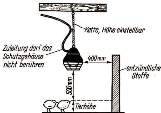
69/4 Beispiel für vorschriftsmäßigen Betrieb eines Infrarotstrahlers
