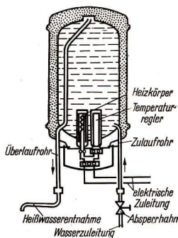
68/1 Schnitt durch einen elektrischen Überlaufspeicher
