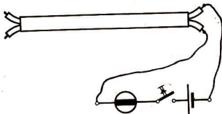
85/5 Prüfen einer Leitung oder eines Kabels auf Kurzschluß mit einem Schauzeichen
