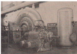
41/4 Wasserturbine
