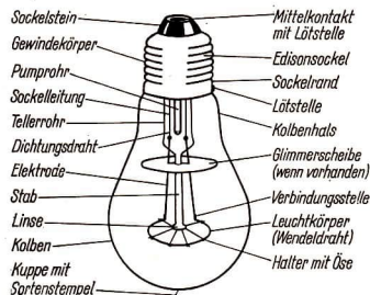
60/1 Glühlampe: Aufbau und Bezeichnungen
