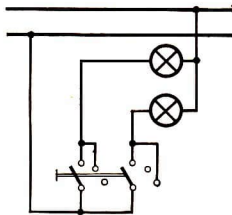
58/2 Serienschaltung
