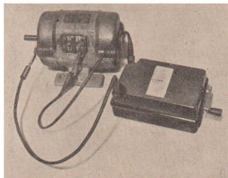
85/4 Prüfen der Wicklungen eines Drehstrommotors auf Körperschluß
