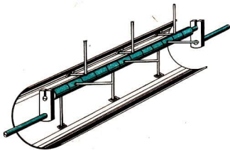
12/1 Befestigung der Exzenterwelle
