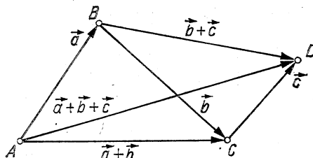
Bild 18 \vec{a} + (\vec{b} + \vec{c}) = (\vec{a} + \vec{b}) + \vec{c} = \vec{a} + \vec{b} + \vec{c}
