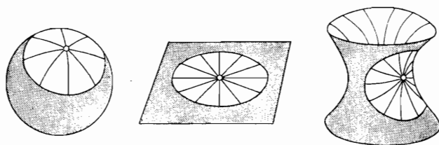
Zweidimensionale euklidische und nichteuklidische Geometrie
