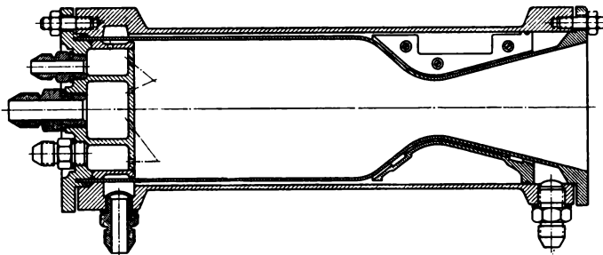
Bild 4.8 Ebener Kammerkopf an zylindrischer Brennkammer
