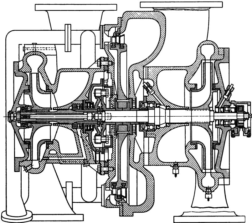
Bild 4.17 Turbopumpenaggregat
