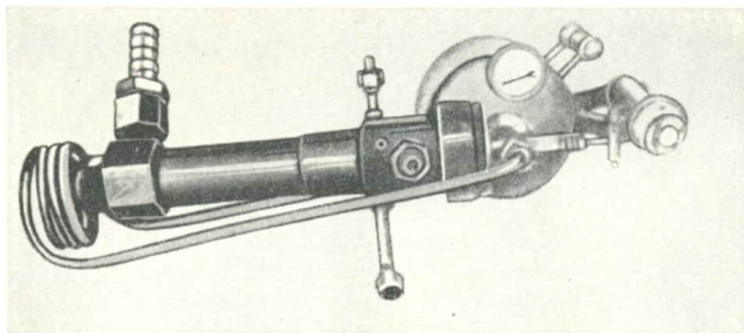
Flüssigkeits-Raketentriebwerk OR-1
