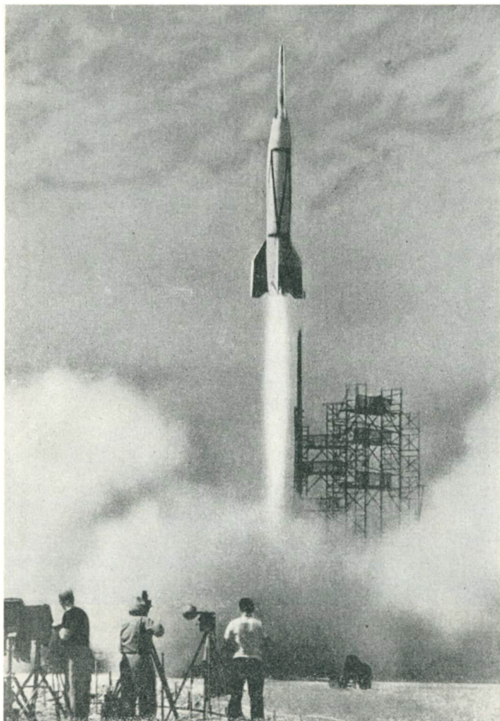
Bild 5.28 Zweistufenrakete Bumper (A4 + WAC-Corporal)
