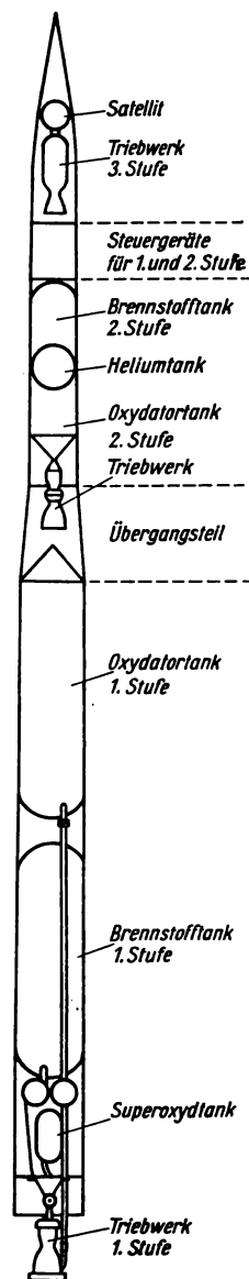
Bild 5.42 Aufbau des Vanguard-Trägersystems
