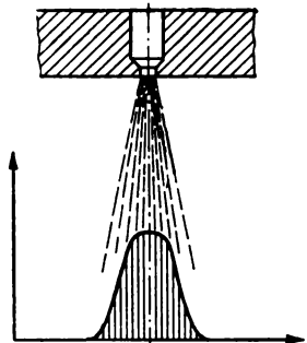
Bild 3.10 Strahlauflösung beim Strahlzerstäuber
