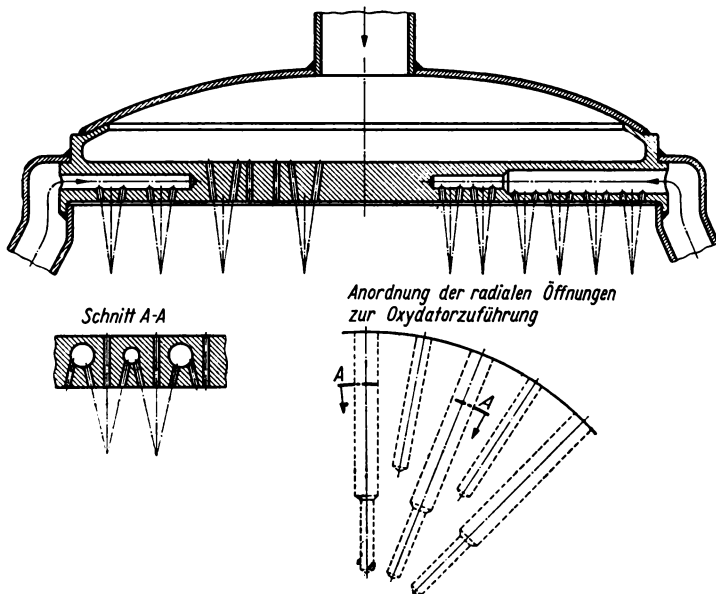
Bild 4.10 Treibstoffzuführung im ebenen Kammerkopf
