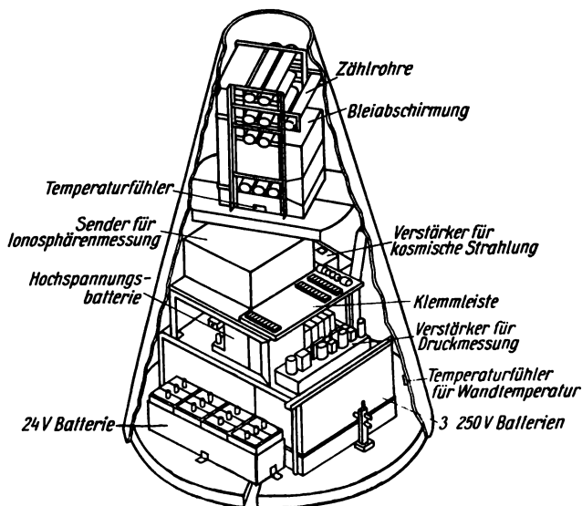
Bild 5.15 Zählrohrteleskop im A4-Meßkopf
