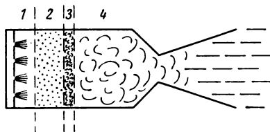
Bild 3.13 Charakteristische Brennkammerbereiche
