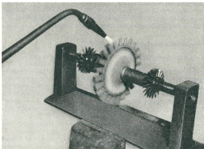
Bild 4.13 Turbinenrad aus WZ-Legierung wird durch ein Knallgasgebläse beaufschlagt (Plansewerk)
