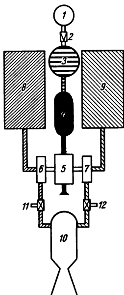
Bild 4.18 Schema der Pumpenförderung
