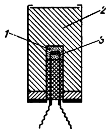
Bild 3.7 Schema eines pyrotechnischen Zünders
