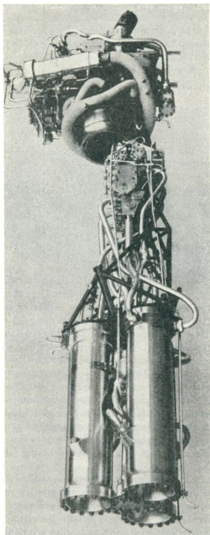
Bild 6.13 Flüssigkeitstriebwerk SEPR 481
