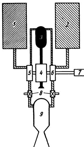
Bild 4.19 Schema der Pumpenförderung unter Verwendung des Haupttreibstoffs
