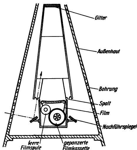
Bild 5.13 Schema eines verbesserten Raketenspektrographen
