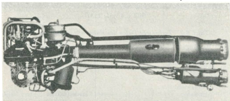
Bild 6.9 Walter-Triebwerk 109-509A1
