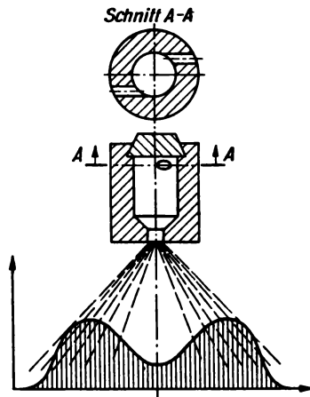
Bild 3.12 Drallzerstäuber
