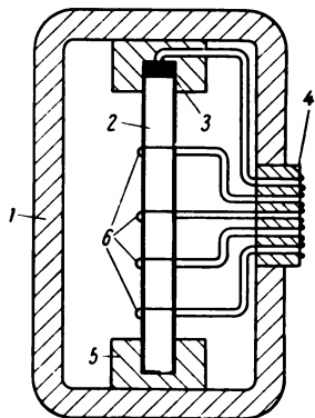
Bild 3.2 Schema einer Meßeinrichtung zur Bestimmung der Verbrennungsgeschwindigkeit v_r fester Treibstoffe
