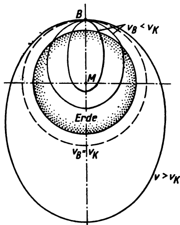
Bild 7.26 Bahnkurven bei einem Abgangswinkel \theta = 0^\circ
