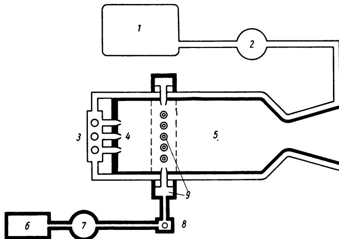
Bild 2.4 Schema eines Atom-Raketentriebwerks vom Mischungstyp
