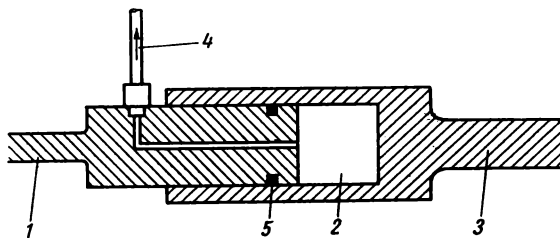
Bild 9.7 Hydraulische Schubübertragung
