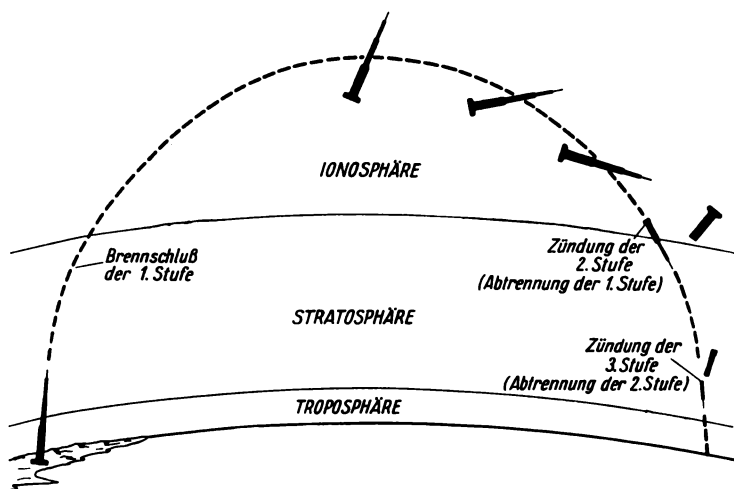
Bild 5.48 Flugweg der X-17
