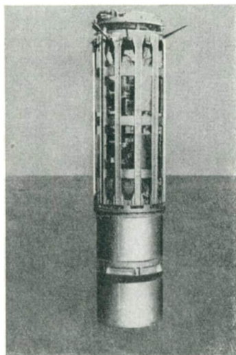
Bild 5.25 Meßgerätebehälter einer sowjetischen Höhenforschungsrakete
