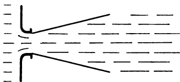
Bild 3.16 Lavaldüse
