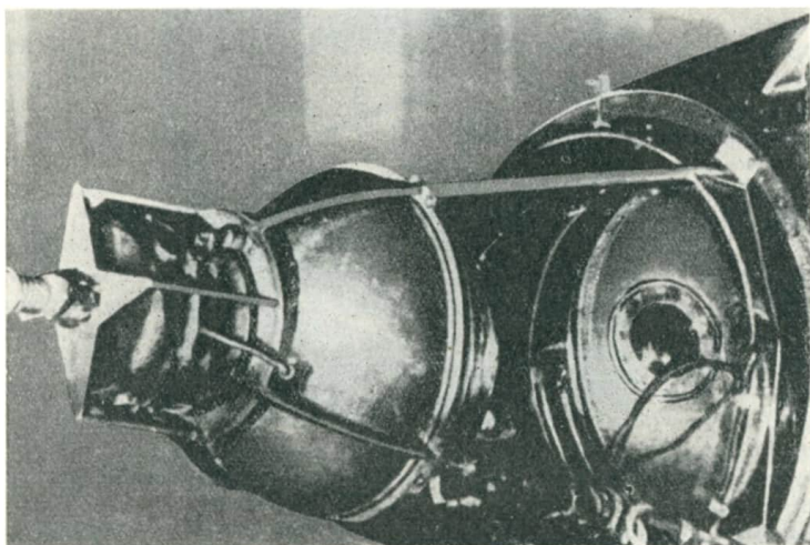
Bild 5.37 Geräteteil des zweiten sowjetischen Satelliten (Sputnik II)
