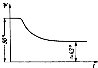
Bild 7.22 Lenkprogramm einer ballistischen Fernrakete
