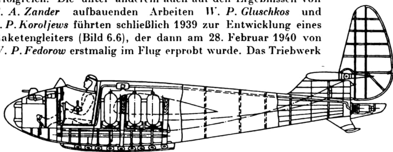
Bild 6.6 Sowjetischer Raketengleiter aus dem Jahre 1940
