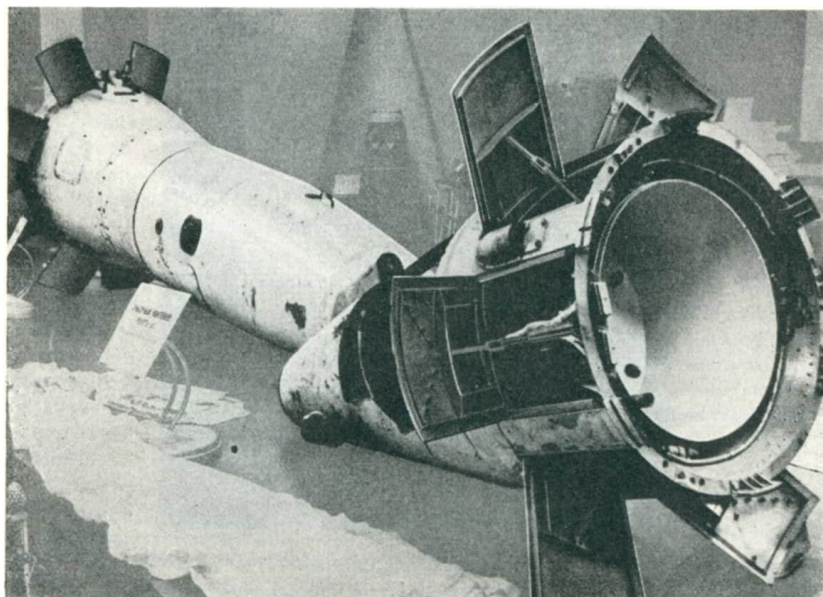
Bild 5.23 Meßkopf einer sowjetischen Höhenrakete vom Typ A 1
