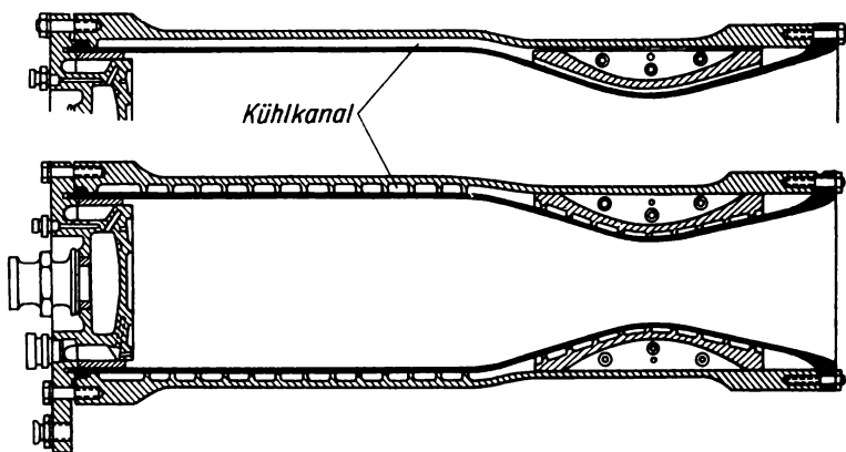
Bild 4.7 Schema einer zylindrischen Brennkammer
