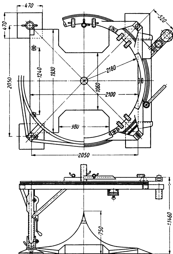
Bild 5.20 Starttisch des A4
