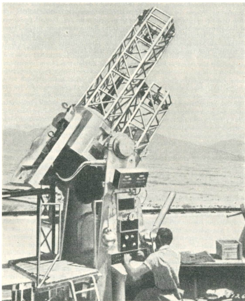
Bild 9.9 Spezial-Spiegelteleskop zur optischen Bahnvermessung
