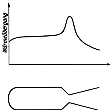
Bild 4.14 Verlauf des Wärmestroms
