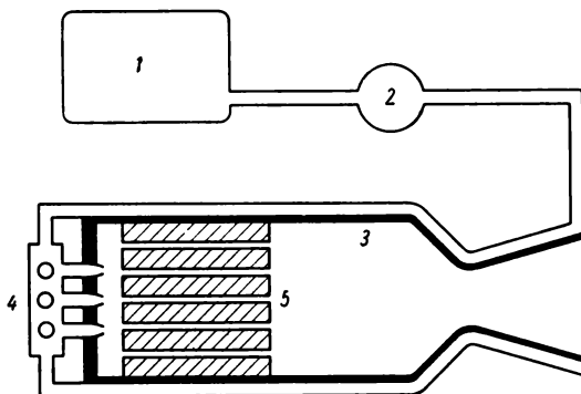
Bild 2.3 Schema eines Atom-Raketentriebwerks vom Reaktortyp
