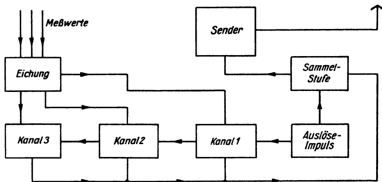
Bild 5.9 Blockschaltbild für einen Meßwertsender
