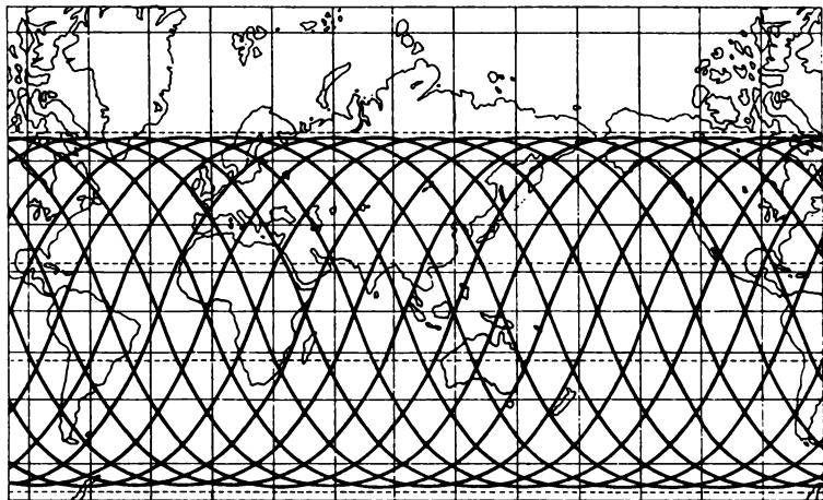
Bild 5.33 Schema der Bahnabwicklung für die ersten sowjetischen Satelliten
