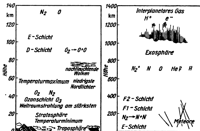
Bild 5.1 Aufbau der Erdatmosphäre
