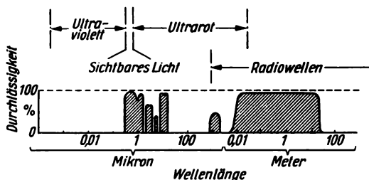
Bild 5.2 Durchlässigkeitsbereiche der Erdatmosphäre
