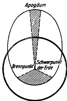
Bild 5.34 Keplerscher Flächensatz
