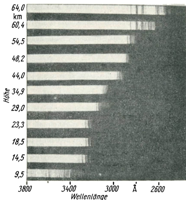
Bild 5.3 Bei einem Raketenanstieg gewonnene UV-Spektren der solaren Strahlung
