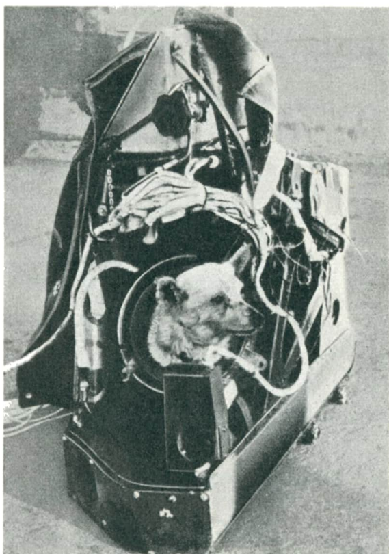
Bild 5.24 Versuchshund in einer Spezialekabinen einer sowjetischen Höhenforschungsrakete
