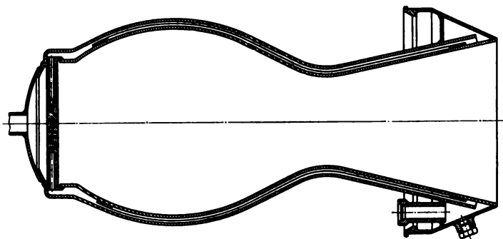
Bild 4.9 Ebener Kammerkopf an birnenförmiger Brennkammer
