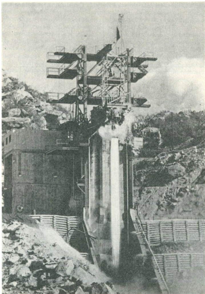
Bild 9.5 Größerer Vertikalprüfstand
