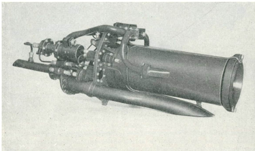
Bild 6.14 Flüssigkeitstriebwerk „Scorpion“ (Napier)
