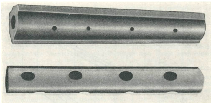
Bild 3.3 Unterbrochener Abbrand eines Treibsatzes
