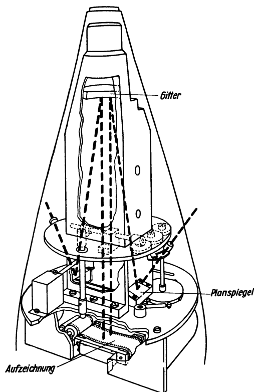
Bild 5.12 Schema eines Raketenspektrographen
