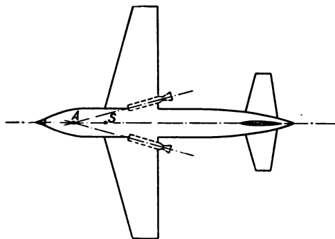
Bild 6.1 Schema der Anordnung von zwei Starthilfen am Flugzeug S Schwerpunkt; A gemeinsamer Angriffspunkt der Rückstoßkräfte
