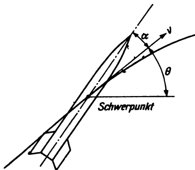
Bild 7.21 Programmwinkel, Bahnwinkel und Anstellwinkel
