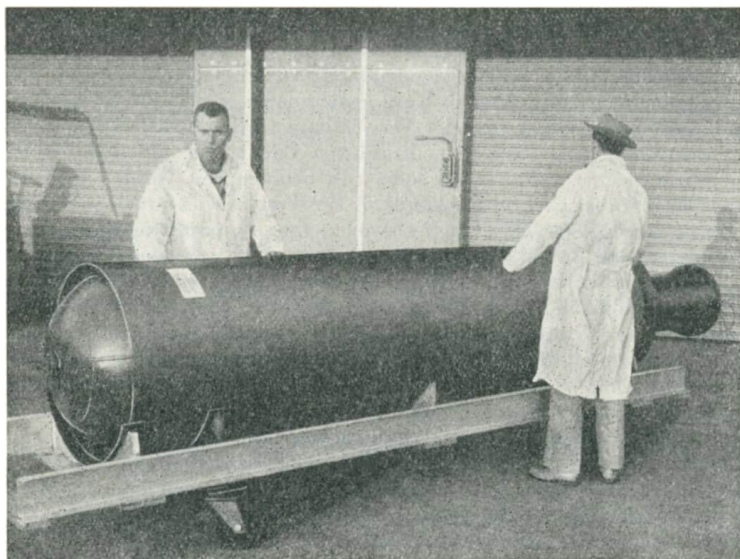
Bild 4.3 Feststofftriebwerk für eine große Feststoffrakete
