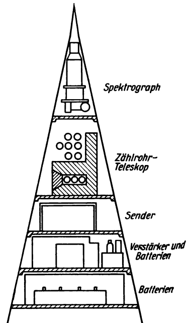
Bild 5.11 Raketen-Meßkopf
