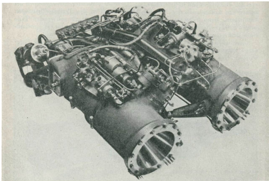
Bild 6.15 Flüssigkeitstriebwerk „Double-Scorpion“ (Napier)
