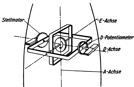
Bild 8.6 Schema des „Horizont“
