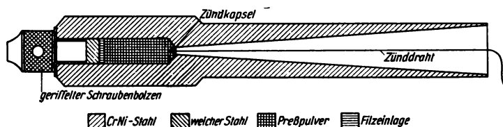
Feststoff-Raketentriebwerk nach R. H. Goddard
