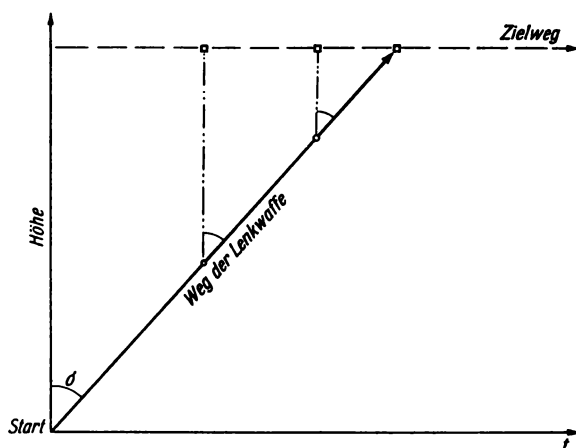
Bild 7.6 Leitstrahlenlenkung mit Vorhaltekurs
