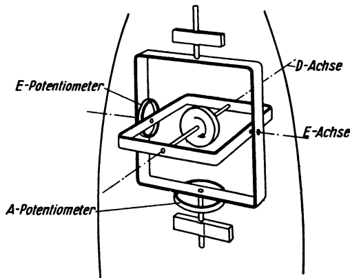
Bild 8.8 Schema des „Vertikant“
