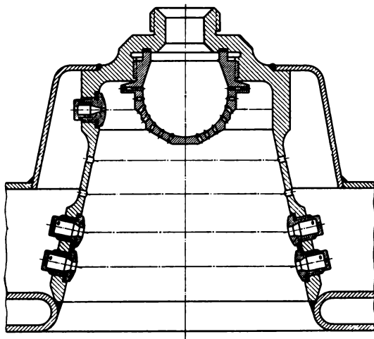
Bild 4.11 Einspritzkopf
