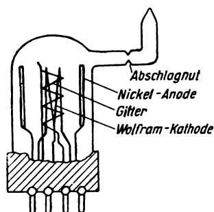
Bild 5.16 Ionisationsvakuummeter
