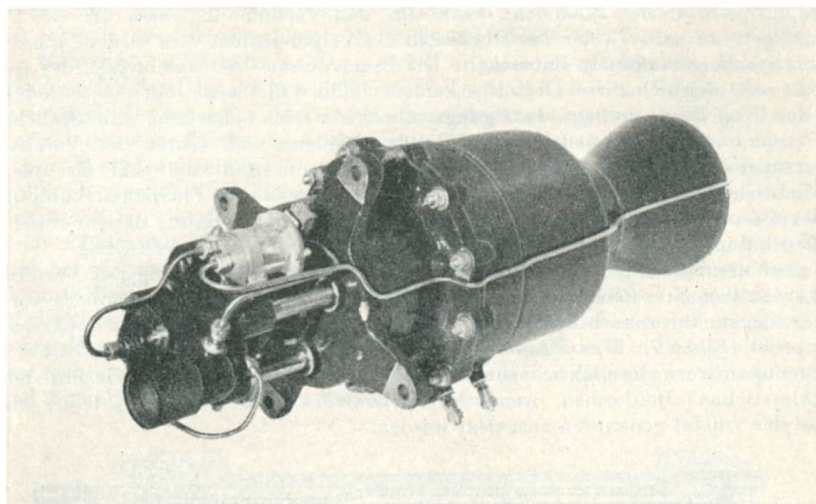
Bild 4.5 Flüssigkeitstriebwerk NER 17 (Napier)
