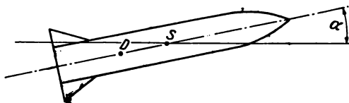
Bild 8.1 Druckmittelpunkt D und Schwerpunkt S , Anstellwinkel \alpha
