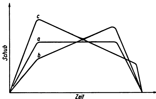
Bild 3.5 Typische Schub-Zeit-Diagramme
