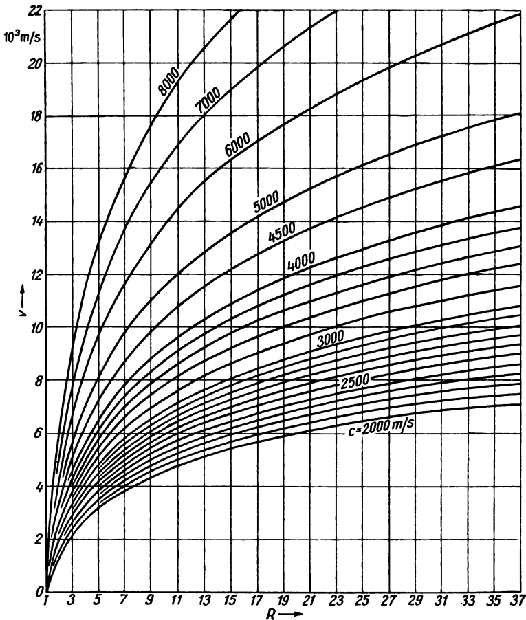
Bild 1.4 Zusammenhang zwischen Massenverhältnis R , Ausströmgeschwindigkeit c und idealer Raketengeschwindigkeit v
