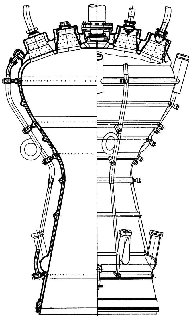
Bild 5.19 A4-Brennkammer
