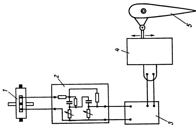
Bild 8.10 Schema des Übertragungsweges Kreisel—Ruder beim A4 1 Krehel; 2 Dämpfungsglied; 3 Verstärker; 4 Rudermaschine; 5 Ruder
