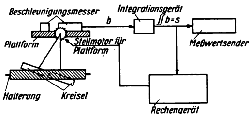
Bild 8.16 Einachsige Plattform
