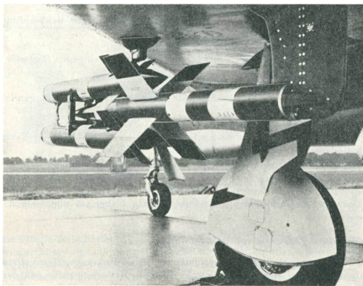
Bild 7.2 „Fireflash“ unter dem Flügel (Fairey)
