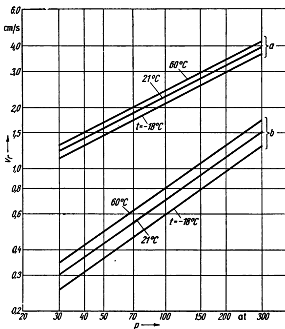
Bild 3.4 Abhängigkeit der Verbrennungsgeschwindigkeit v , vom Druck p und von der Anfangstemperatur t
