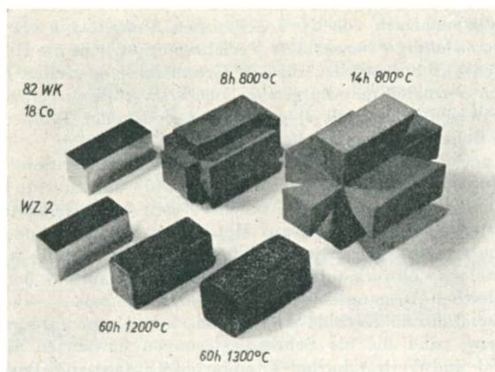
Bild 4.12 WZ-Legierungen nach verschiedenen Temperaturtests (Planseewerk)
