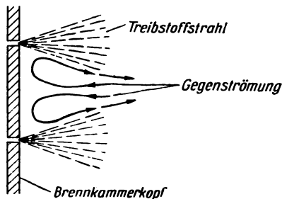
Bild 3.8 Gegenströmung zwischen den Einspritzstrahlen
