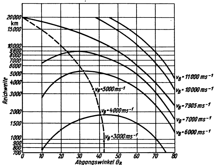
Bild 7.28 Abhängigkeit der Reichweite von Abgangswinkel und Brennschlußgeschwindigkeit
