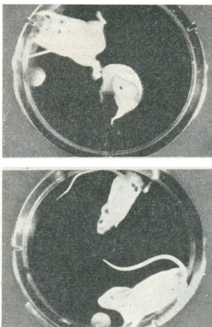
Bild 5.6 In einer Trommelkammer eingeschlossene Mäuse während eines Raketen- aufstiegs
