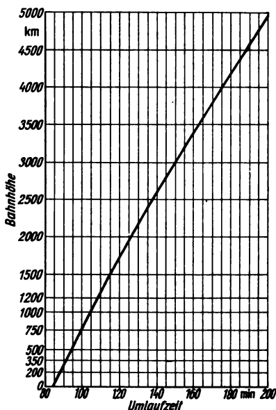
Bild 5.31 Beziehung zwischen Umlaufzeit t_K und Kreishöhe H
