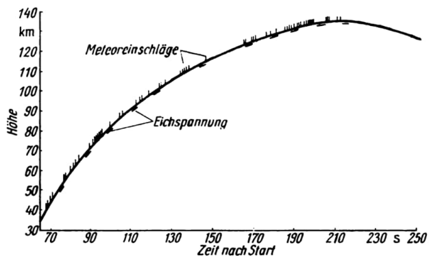
Bild 5.7 Registrierkurve von Treffern durch Mikrometeore mit Meßmarken
