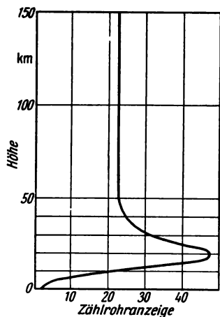
Bild 5.4 Änderung der Intensität der primären Ultrastrahlung mit der Höhe
