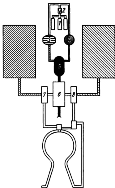
Bild 4.20 Förderschema des A4
