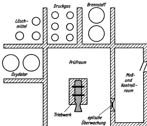
Bild 9.3 Aufbauschema eines Horizontalprüfstands
