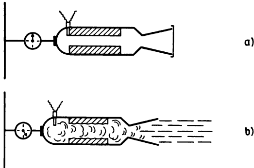
Bild 1.2 Vereinfachtes Funktionsschema eines Raketentriebwerks
