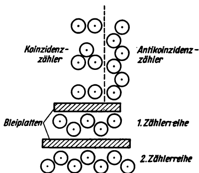
Bild 5.14 Aufbau eines Zählrohrteleskops (schematisch)
