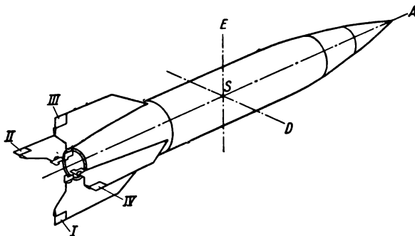
Bild 8.5 Achsen und Anordnung der Ruder beim A4
