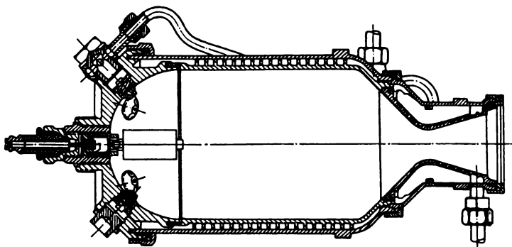
Bild 6.7 Brennkammer des Triebwerks des sowjetischen Raketenfliegers
