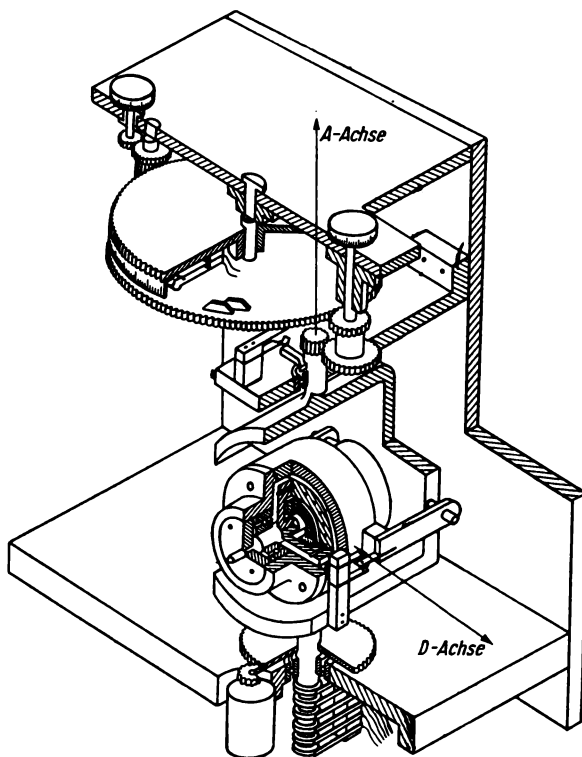
Bild 8.12 Kreiselintegrator
