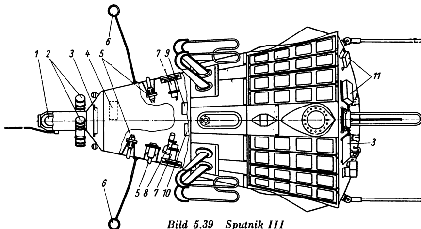
Bild 5.39 Sputnik III
