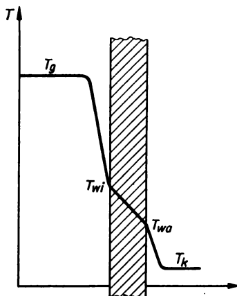
Bild 4.15 Wärmedurchgang durch Brennkammerwand
