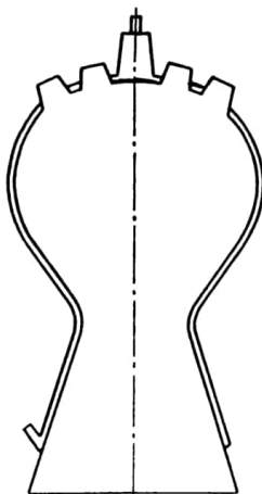
Bild 4.6 Schema einer kugelförmigen Brennkammer
