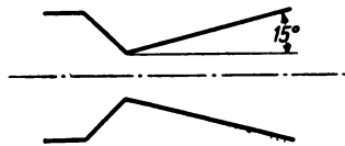
Bild 3.18 Düsenöffnungswinkel
