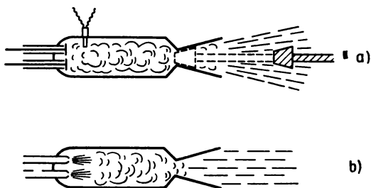
Bild 1.3 Wechseldruck- und Gleichdruck-Raketentriebwerk
