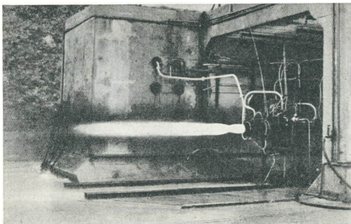
Bild 9.1 Kleinerer Horizontalprüfstand
