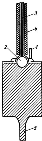
Bild 9.8 Prinzip des induktiven Schwimmer-Mengenmessers
