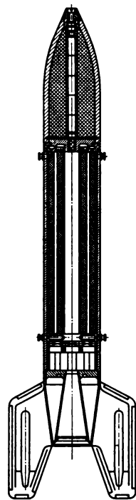
Bild 4.4 Feststoffrakete mit Stabilisierungsflossen
