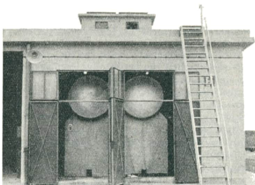
Bild 9.2 Treibstoffbehälter in separaten Boxen
