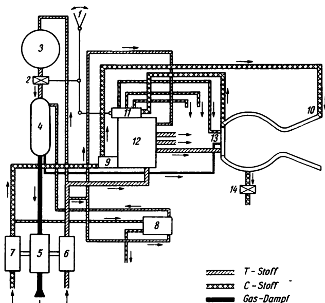
Bild 6.10 Betriebsschema des Walter-Triebwerks 109-509A1
