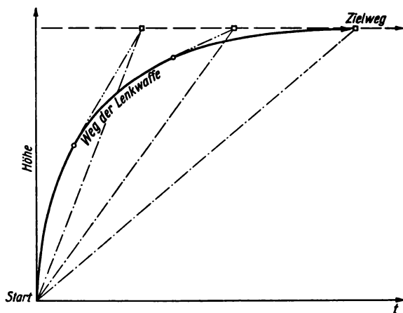
Bild 7.7 Leitstrahlenlenkung auf Hundekurve
