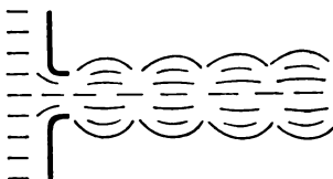
Bild 3.15 Strahlausbreitung hinter einer konvergenten Düse
