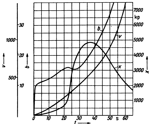
Bild 7.25 Änderungen von Geschwindigkeit, Beschleunigung und Stirnwiderstand beim A4
