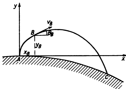
Bild 7.20 Koordinaten des Brennschlußpunktes und Abgangswinkel
