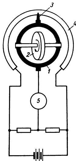
Bild 8.4 Schema einer einfachen Kurssteuerung
