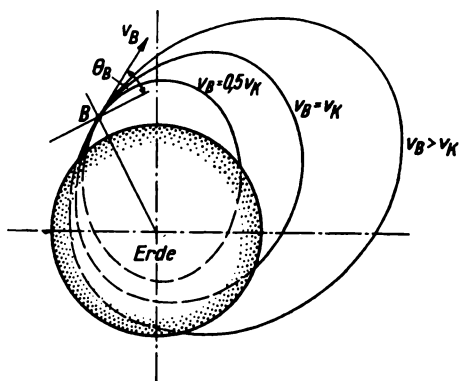
Bild 7.27 Bahnkurven bei \theta = 30^\circ
