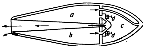
Sauerstoff-Wasserstoff-Rakete nach Ziolkowski
