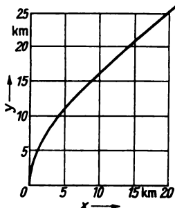
Bild 7.24 Aktiver Bahnabschnitt (Antriebsstrecke) einer ballistischen Fernrakete
