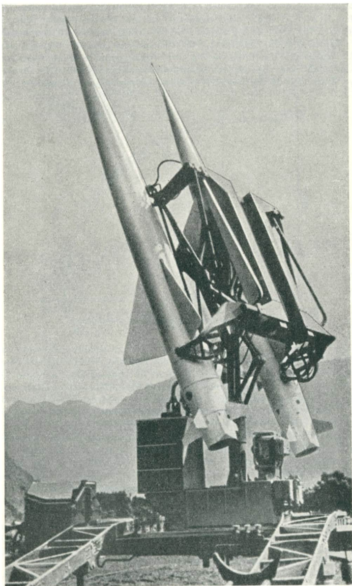
Bild 7.5 Oerlikon-Flabrakete 54 in Doppellafette
