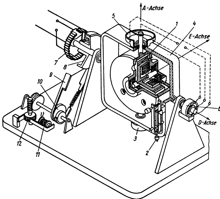
Bild 8.7 „Horizont“ der A4-Steuerung
