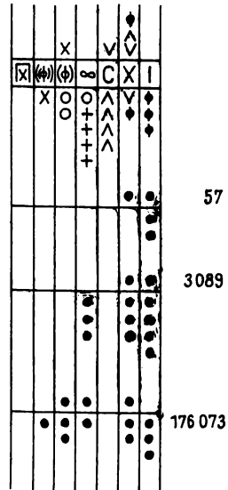
Bild 8. Darstellung der Multiplikation auf dem Abakus
