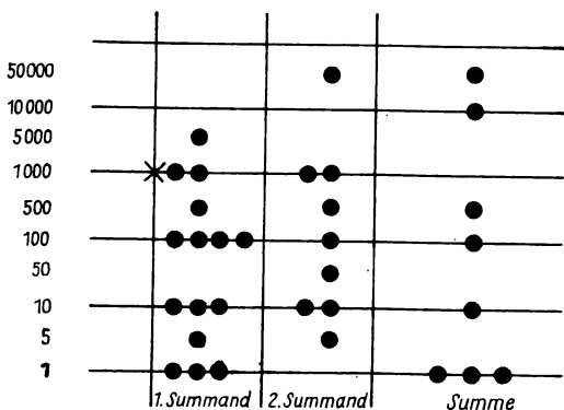
Bild 23. Darstellung einer Addition auf dem Abakus
