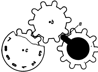
Bild 34. Das Prinzip des Vermittlungsradsystems (schematisch)
