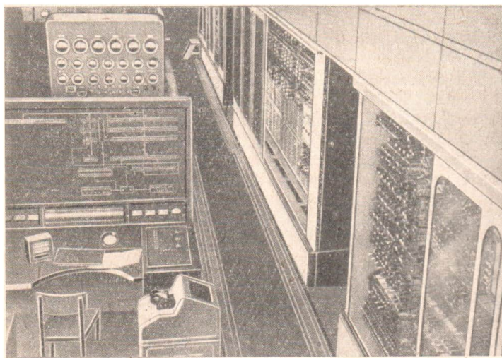
Bild 41. Sowjetischer Digitalrechner sehr hoher Leistungsfähigkeit (BESM)
