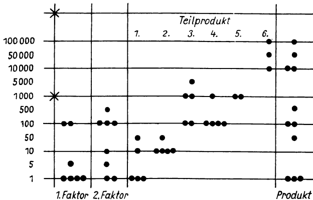
Bild 25. Darstellung einer Multiplikation auf dem Abakus
