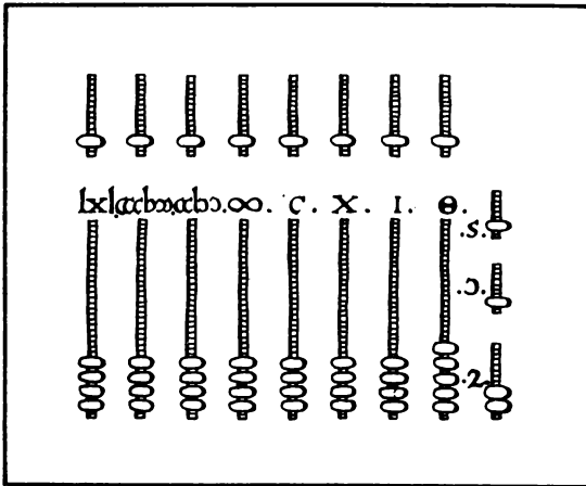
Bild 6. Römischer Abakus
