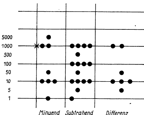
Bild 24. Darstellung einer Subtraktion auf dem Abakus
