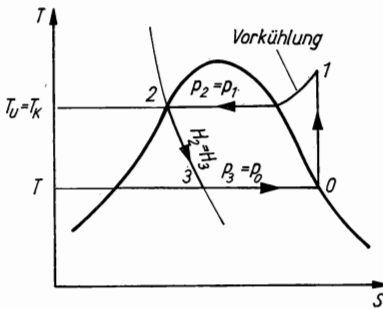
Bild 2.2.10. T,S -Diagramm des Kühlprozesses
