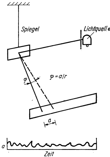
Bild 1.3.3. Nullpunktschwankungen eines Drehspeiegels
