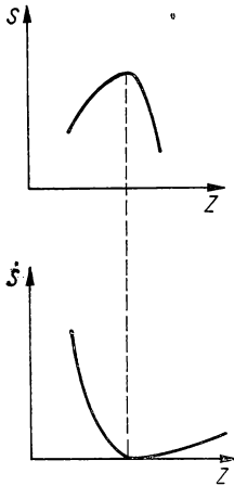
Bild 3.2.1. Entropie S und Entropieproduktion P in der Nähe des thermodynamischen Gleichgewichtszustandes
