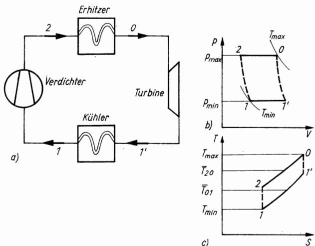
Bild 1.2.7. Gasturbinenanlage im JOULE-Prozeß a) Schaltschema, b) p, V -Diagramm, c) T, S -Diagramm
