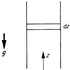
Bild 1.3.2. Luftsäule
