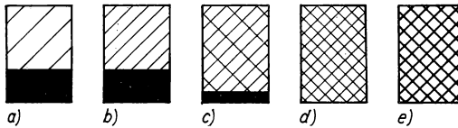
Bild 2.2.2. Gleichgewichtszustände des Wassers und seines Dampfes ( x Dampfanteil)
