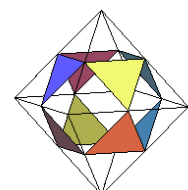
Oktaeder ergibt ein Kuboktaeder
