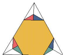
Tetraeder ergibt für k = 1/3 ein abgestumpftes
