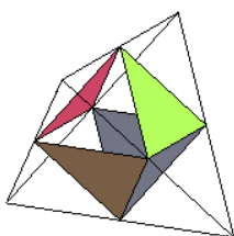
Tetraeder ergibt ein regelmäßiges Oktaeder
