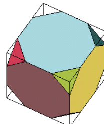
Würfel ergibt für k = 1/(2+\sqrt{2}) einen abgestumpften
