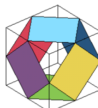
Würfel ergibt ein Kuboktaeder
