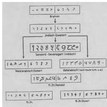
7 Schreibweise der indisch-arabischen Ziffern in ihrer historischen Entwicklung. Nach K.Menninger
