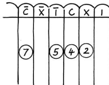
8 Rechenbrett des Gerbert von Aurillac, 10.Jh. Die Linien sind senkrecht. Verwendet werden Rechensteine, die indische Ziffern tragen (sog. Apices). Prinzipskizze. Aufgelegt ist die Zahl 705420. Nach K.Menninger
