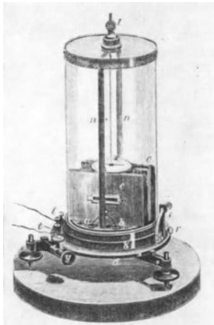
4 Multiplikator (In: Cyon, E.: Atlas zur Methodik der physiologischen Experimente und Vivisektionen. Gießen 1876. Tafel XXXIX. Abb.3.)
