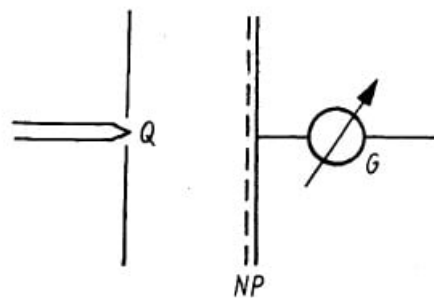
7 Anordnung zur Untersuchung der Energieverluste bei Zusammenstößen zwischen Elektronen und Atomen [46]
