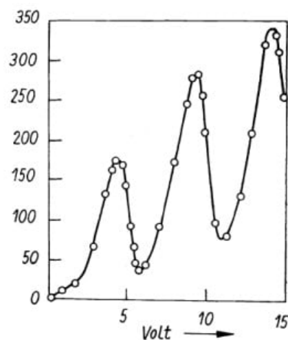
8 Strom zur Auffangplatte in Abhängigkeit von der die Elektronen beschleunigenden Spannung, gemessen in Quecksilberdampf mit einer Gegenspannung von 0,1 V [46]
