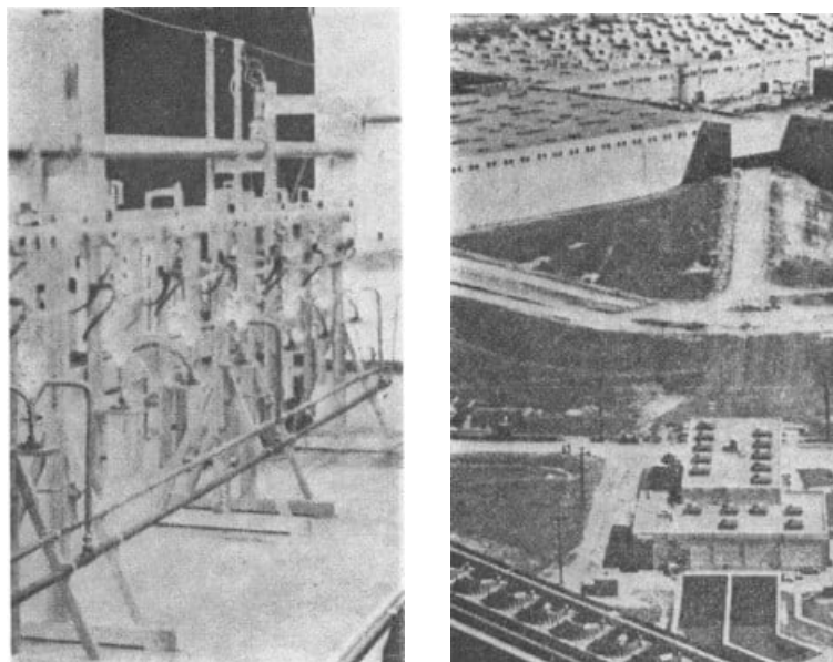
11 Die von Gustav Hertz 1934 gebaute Diffusionskaskade zur Isotopentrennung im Laboratorium der Technischen Hochschule Berlin-Charlottenburg [48] und ...
