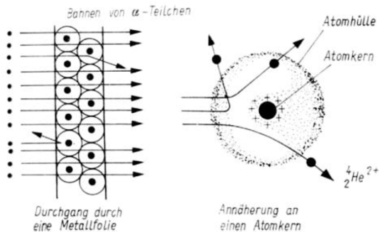
5 Bahnen von Alpha-Teilchen
