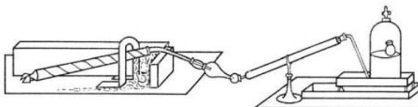
9 Apparatur zur organischen Elementaranalyse nach Berzelius (nach [44]).
