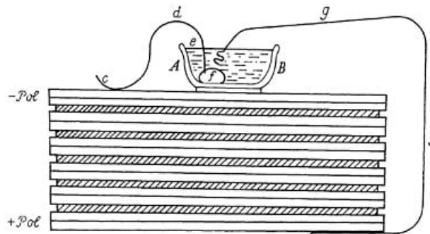
7 Anordnung zur Elektrolyse mit einer Quecksilberkathode (f) zur Abscheidung von Alkalimetallen nach Berzelius und Pontin (aus [B 12]).
