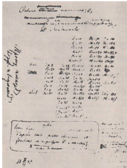
Abb. 3. Faksimileausschnitt eines handschriftlichen Entwurfs Mendelejews für das Periodensystem (vom 17. 2. 1869)
