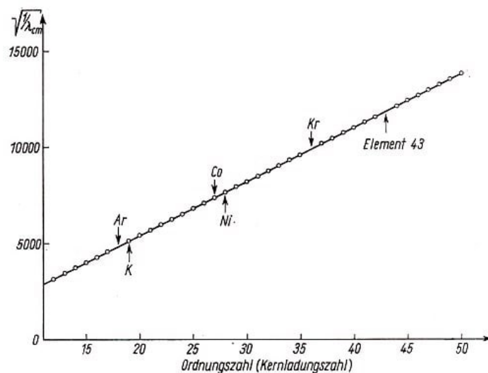
Abb. 6. Graphische Darstellung des Moseleyschen Gesetzes
