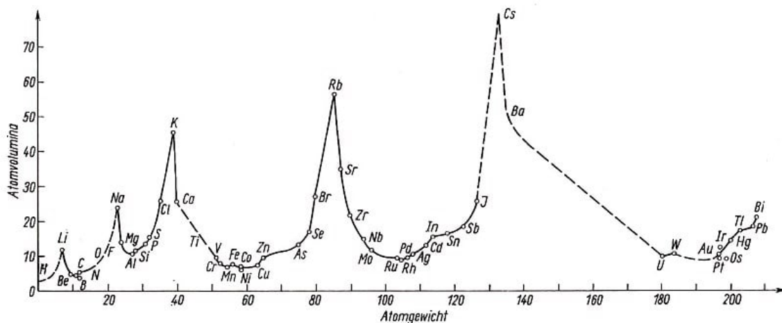
Abb. 4. Atomvolumenkurve Lothar Meyers
