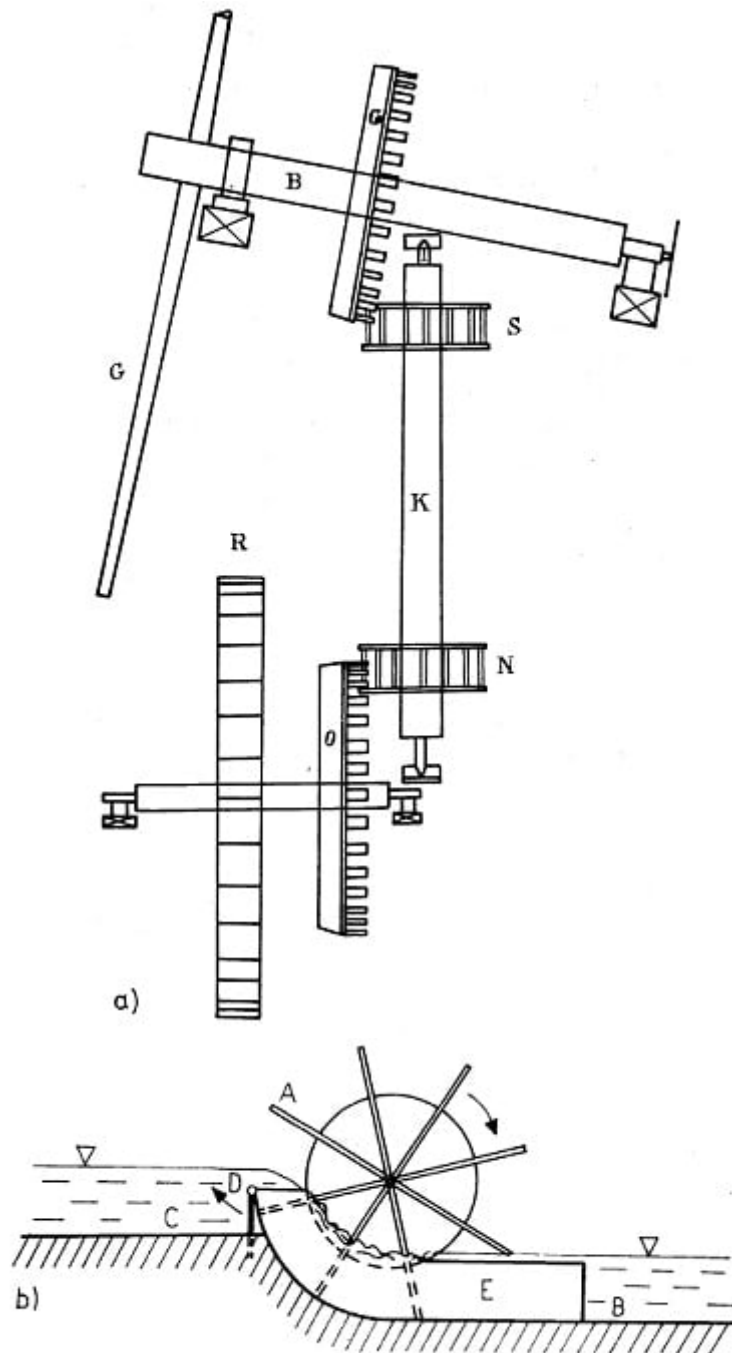
22 Schema einer windgetriebenen Entwässerungsmühle (Ende des 16. Jahrhunderts)
