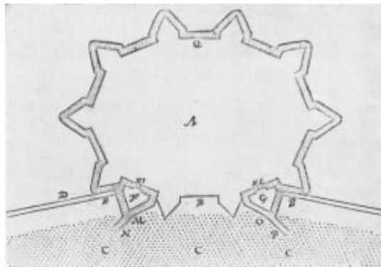
28 Vorschlag für die zusätzliche Befestigung einer am Meer gelegenen Stadt durch einen Wasserkanal. KL und HT sind Schleusen (Kammer- und Spülschleusen), G und F Bastionen zu deren Schutz [17]
