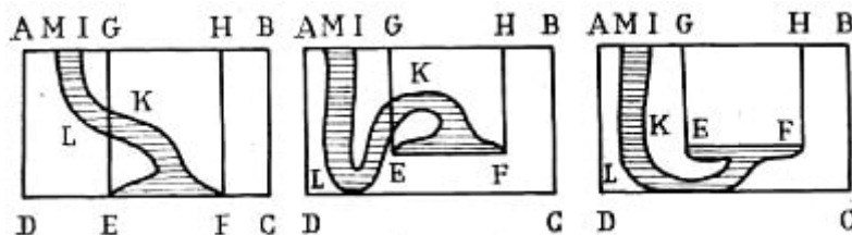
17 Hydrostatisches Paradoxon: Die auf die Fläche EF wirkende Kraft ist stets gleich dem Gewicht einer Wassermenge EFHG [9]
