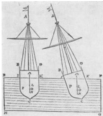
31 Zur Schwimmelage eines Schiffes. O Schwerpunkt des Schiffes, L Angriffspunkt des Auftriebs [14] Kräftedreieck [14]
