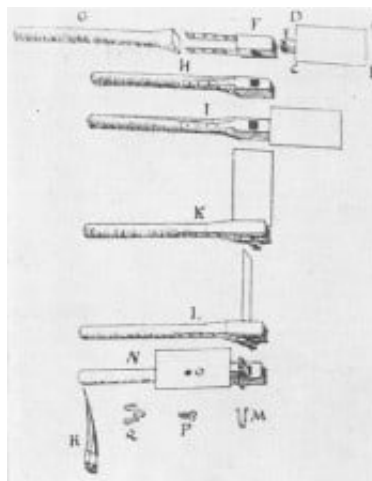
29 "Spabijlkou", Verwendung als Spaten (Spa), K als Beil (bijl), L als Hacke (hou), N im Transportzustand. Oben und unten sind die Einzelteile gezeichnet [21e, S. 477]
