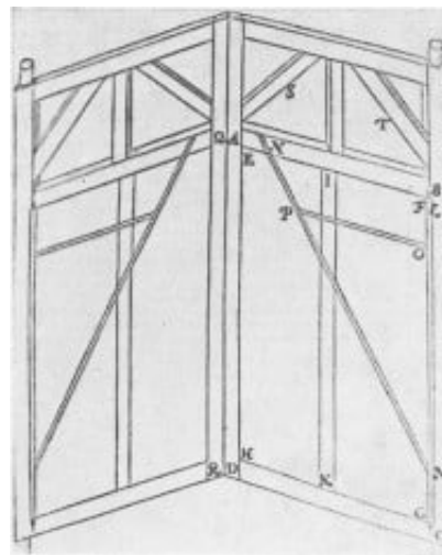
24 Schema eines Schleusentores, das wahlweise zum Betrieb einer Kammer- oder Spülschleuse benutzt werden kann [17]
