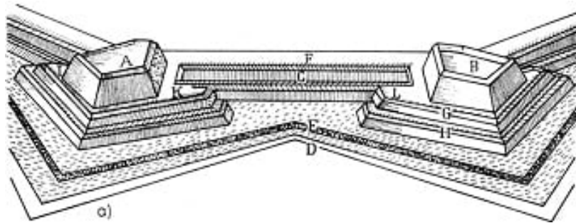
27 a) Perspektivische Ansicht zweier Bastionen und einer Kurtine [12]
