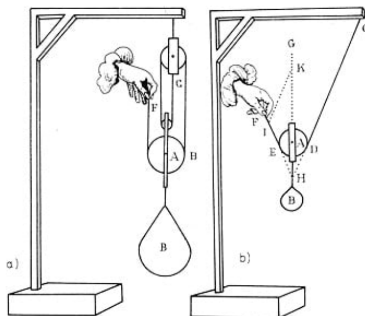
30 a) Flaschenzug mit paralleler Seilführung [14]
