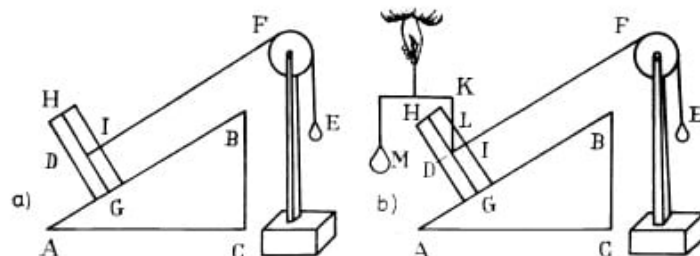
8a Der Körper D wird durch das Gewicht des Körpers E im Gleichgewicht gehalten [7]
