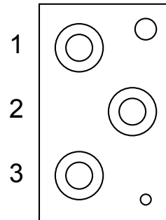
BUCHSENLEISTE 428-3 TGL 29331/07-1
