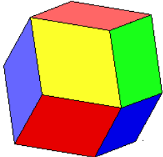
Rhombendodekaeder
