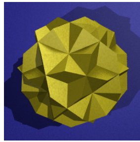
Ikosaeder Sternkörper S4
