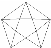
Fünfseitiges Antiprisma
