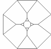
Abgeschnittene r Würfel
