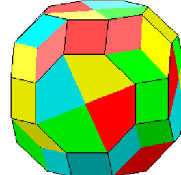
Großes Rhombenkuboktaeder
