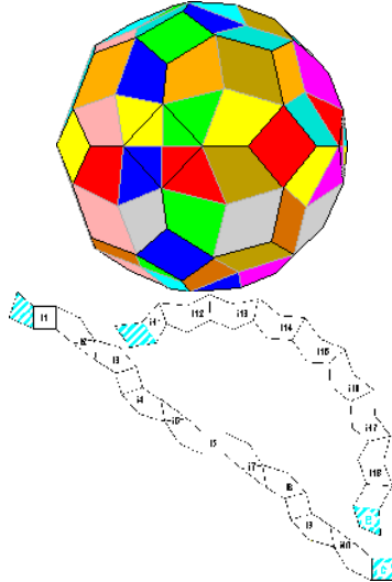
t4-abgestumpftes Deltoid-Ikositetraeder
