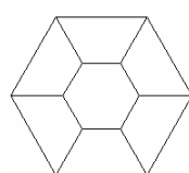
Sechseitiges Prisma
