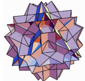
Großes Rhomben-Dodekaeder uniformes Polyeder U_{73} Umkugelradius für Kantenlänge a : R = 1/2 \sqrt{(11 - 4\sqrt{5})} a \approx 0.716890 a
