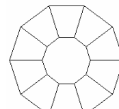
Zehnseitiges Prisma
