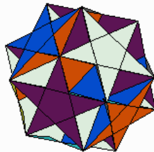
Ditrigonales Dodekadodekaeder auch ditrigonales Dodekaeder genannt uniformes Polyeder U_{41} Wythoff Symbol 3 \ | \ 5/3 \ 5 für Kantenlänge a wird der Umkugelradius zu: 1/2 \sqrt{3} a \approx 0.866025 a
