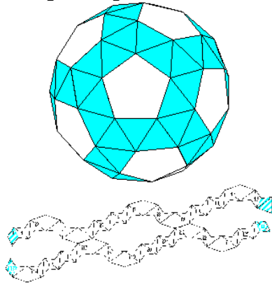
Abgeschrägtes Dodekaeder
