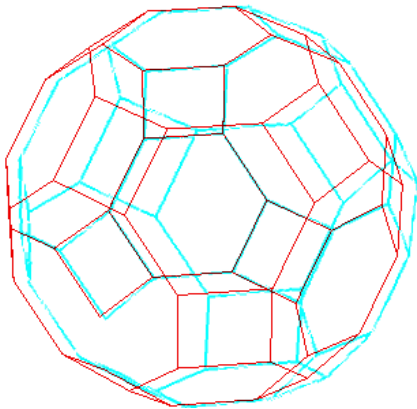
Abgeschnittener Rhombenkuboktaeder
