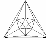
Iksaeder
