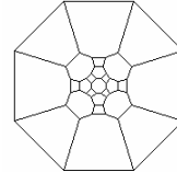
Abgeschnittenes Rhomben- kuboktaeder
