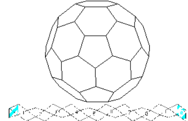
Abgestumpftes Ikosaeder
