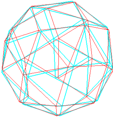
Abgeschrägter Würfel
