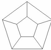
Fünfseitiges Prisma
