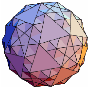
Kleines abgeschnittenes Ikosidodekaeder Das uniforme Polyeder U_{32} , welches dual zum Kleinen hexagonalen Hexacontaeder ist, besitzt das Wythoff Symbol | 3 \ 3 \ 5/2 . Für eine Kantenlänge von a beträgt der Umkugelradius: R = 1/4 \sqrt{(13 + 3\sqrt{5} + \sqrt{(102 + 46\sqrt{5})})} a \approx 1.45819033 a
