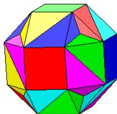
Rhombenkuboktaeder
