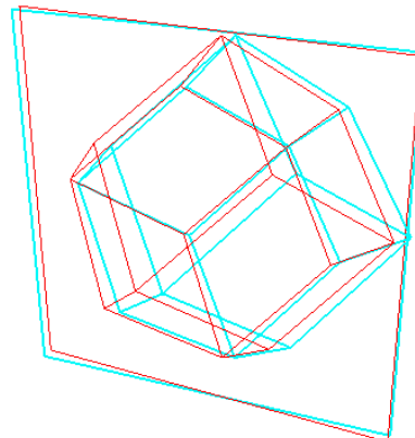
Rhombendodekaeder
