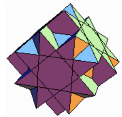
Großes Kuben-Kuboktaeder uniformes Polyeder U_{14} , welches dual zum Großen Hexacronic-Ikositetraeder ist. Wythoff Symbol 34 \ | \ 4/3 Umkugelradius für Kantenlänge a : R = 1/2 \sqrt{(5-2\sqrt{2})} a \approx 0.736812 a , die konvexe Hülle des Polyeders ist der Archimedische Körper A_9 , der abgestumpfte Hexaeder
