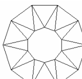
Zehnseitiges Antiprisma
