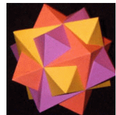
Kantenlängen
