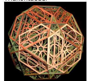
Kleines Dodekaikosaeder
