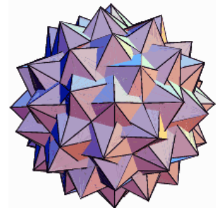
Großes Stern Dodekaikosidodekaeder uniformes Polyeder U_{64} Umkugelradius für 1 Einheit Kantenlänge R = 1/2 \sqrt{2}
