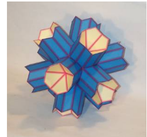
Rhombisches Triakontaeder
