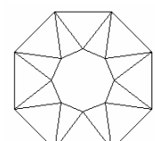
Achtseitiges Antiprisma
