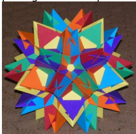
Verbund von 6 Pentagramm Antiprismen
