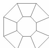
Achtseitiges Prisma
