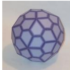
Pentagonaler Hexakontaeder
