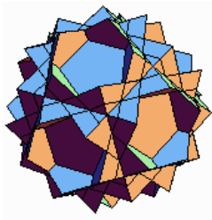
Kleines abgeschnittenes Sterndodekaeder uniformes Polyeder U_{58} Polyeder ist dual zum Großen Pentakis-Dodekaeder Umkugelradius für Kantenlänge a : R = 1/4 \sqrt{(34 - 10\sqrt{5})} a \approx 0.852911 a
