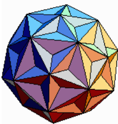
Dodekaeder-kleines Icosaeder-Verbund Sternpolyeder, bei Konstruktion aus einem Dodekaeder; mit Kantenlänge a ergibt sich das Volumen dieses Körpers zu Volumen V = 1/20 (35 + 15\sqrt{15} - 4\sqrt{(10(65 - 29\sqrt{5}))}) a^3 \approx 4.40651 a^3
