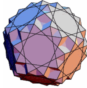
Großes abgeschnittenes Dodekaeder auch Großes dodekaedrisches Icosaeder genannt Das uniforme Polyeder U_{63} , welches dual zum Großen ditrigonalen Dodeka-Hexacontaeder ist, besitzt das Wythoff Symbol 3 \ 5 \ | \ 5/3 . Für eine Kantenlänge von a beträgt der Umkugelradius: R = 1/4 \sqrt{(34 - 6\sqrt{5})} a \approx 1.13422 a Die konvexe Hülle des Polyeders ist ein Pentagondodekaeder.
