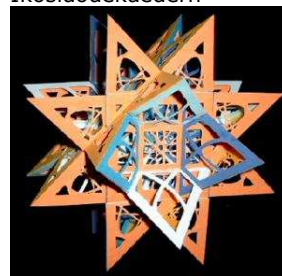
Sternförmiger abgeschnittener Würfel
