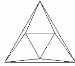
Oktaeder
