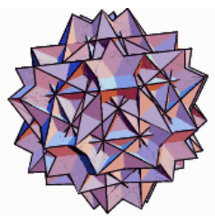
Großes Rhombenikosidodekaeder uniformes Polyeder U_{67} auch Quasi-Rhombenikosidodekaeder genannt, Polyeder ist dual zum Großen Deltoid-Hexcontaeder Umkugelradius für Kantenlänge a : R = 1/2 \sqrt{(11 - 4\sqrt{5})} a \approx 0.716890 a
