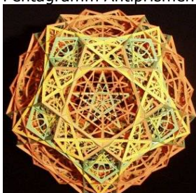
Großes Ikosikosidodekaeder
