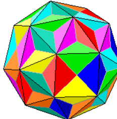
Abgeschrägter Würfel
