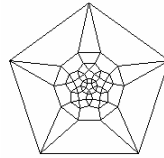
Rhomben- ikosidodekaede r
