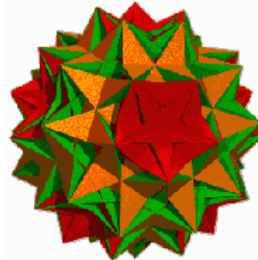
Großes Dirhomben-Ikosidodekaeder uniformes Polyeder U_{75} Umkugelradius für 1 Einheit Kantenlänge R = 1/2 \sqrt{2}
